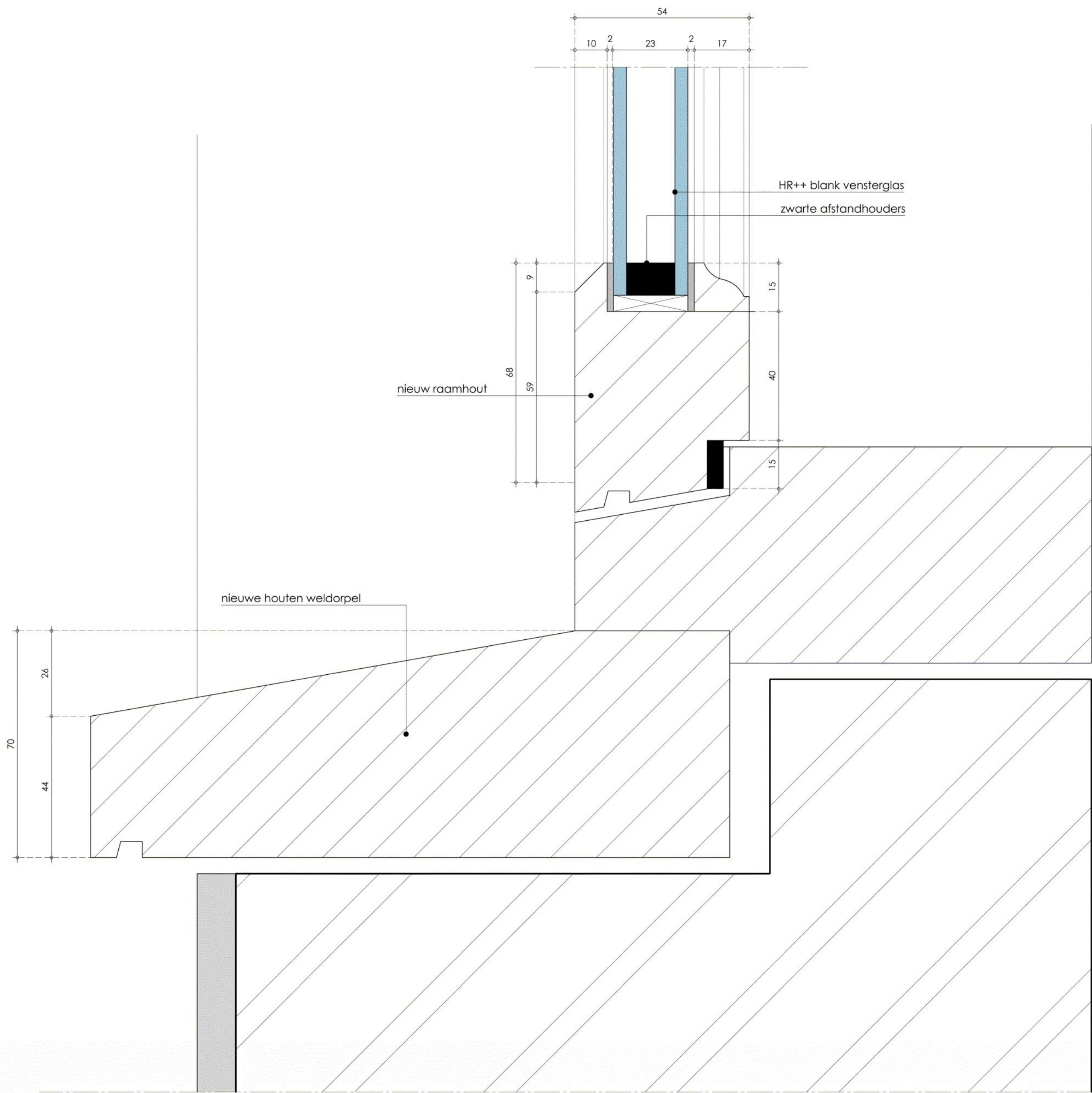
detail 2 nieuwe toestand
