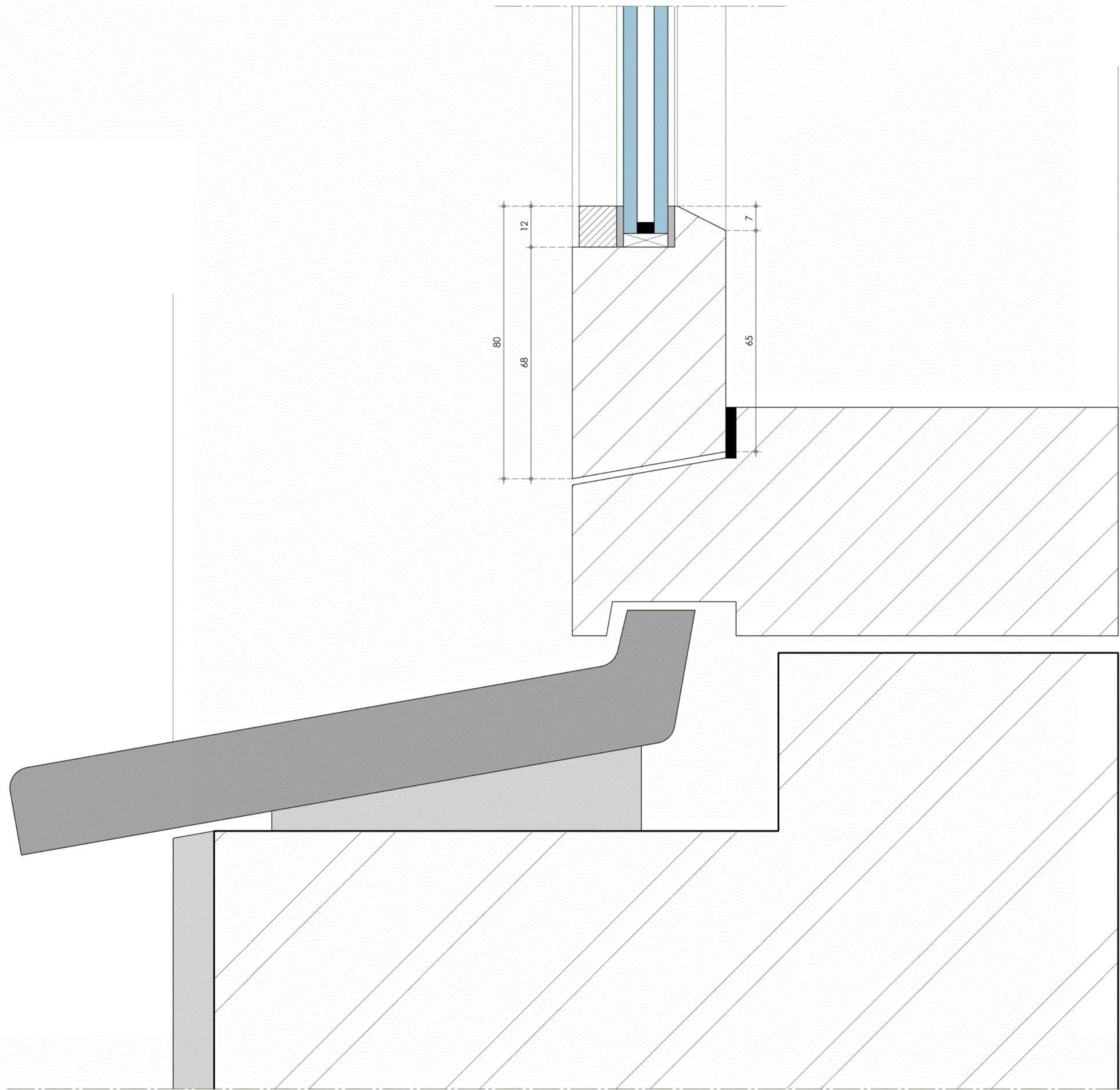
detail 2 bestaande toestand
