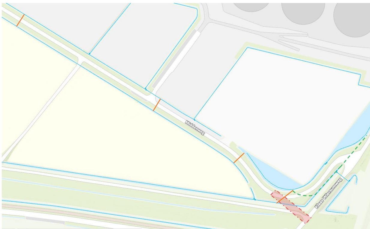
Figuur 1: Nieuwe duikers zijn weergegeven met oranje lijnen, de nieuwe wegaansluiting (inclusief slootdemping) is weergegeven met het rode vlak, de nieuw te graven watergang en her te profileren bestaande watergang zijn weergegeven met groene stippellijn.
