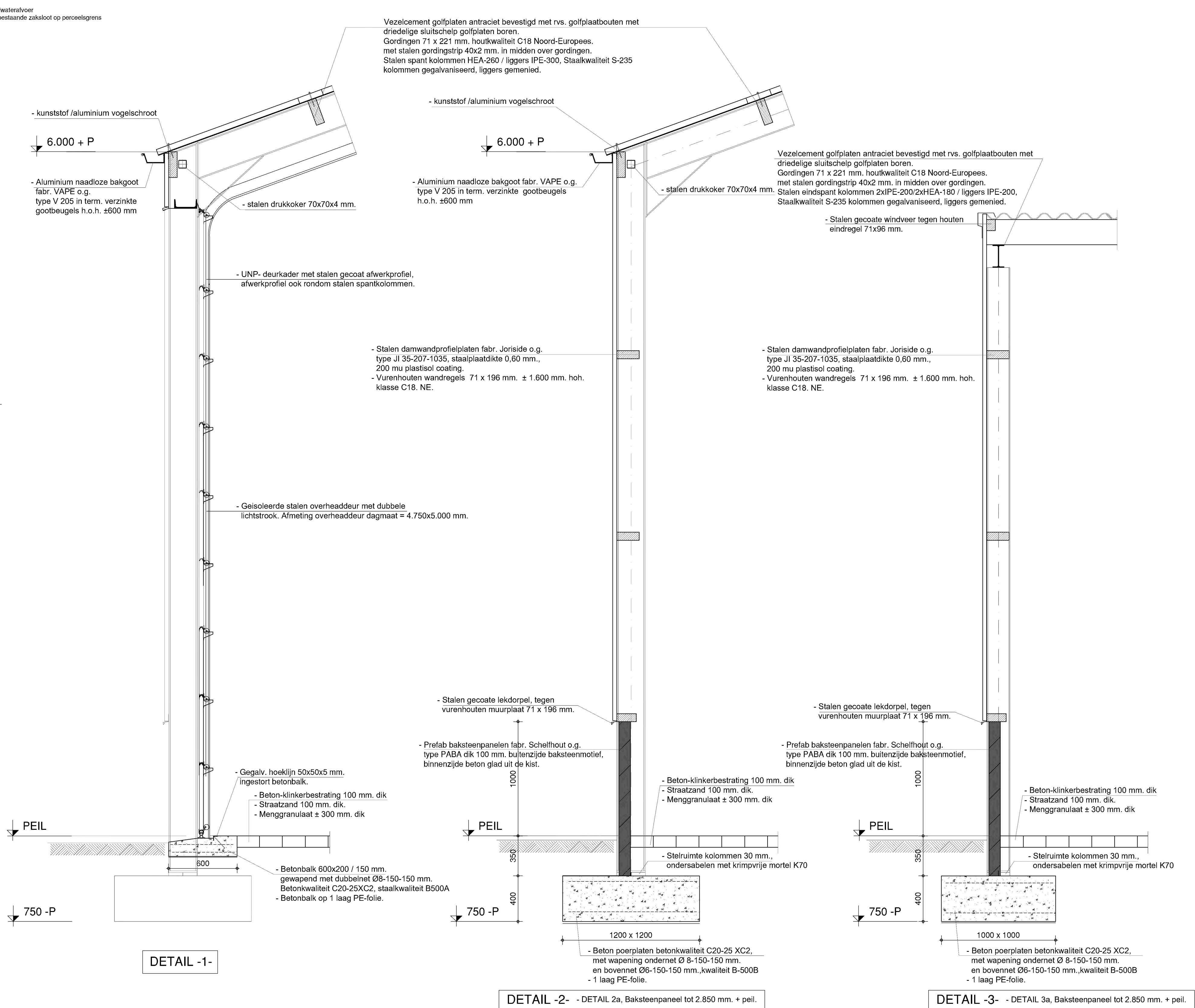
DETAIL -2- - DETAIL 2a, Baksteenpaneel tot 2.850 mm. + peil.
