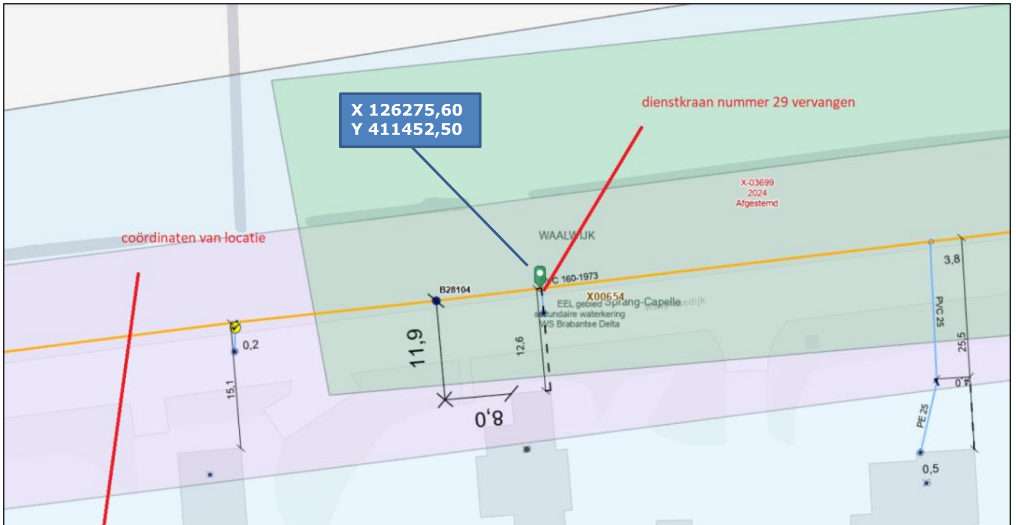
678862-B situatietekening
