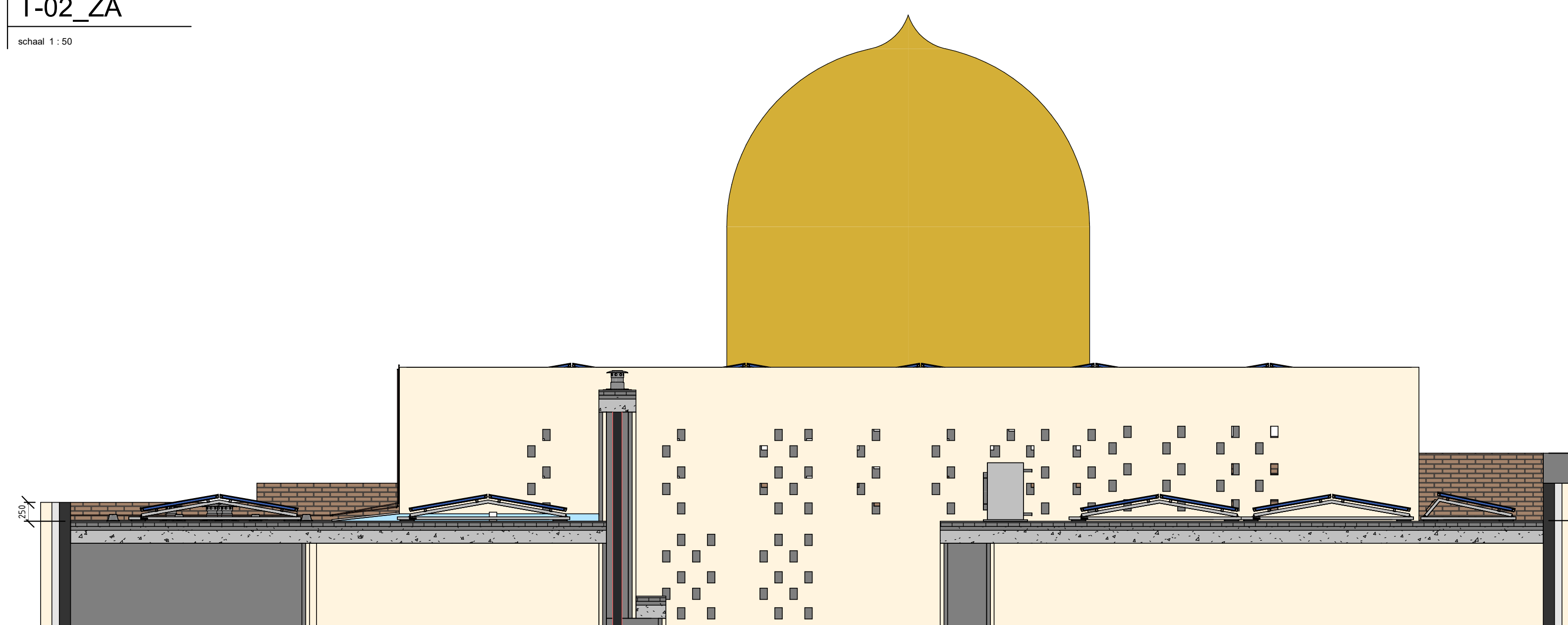
3 | T-02_VA schaal 1:50
