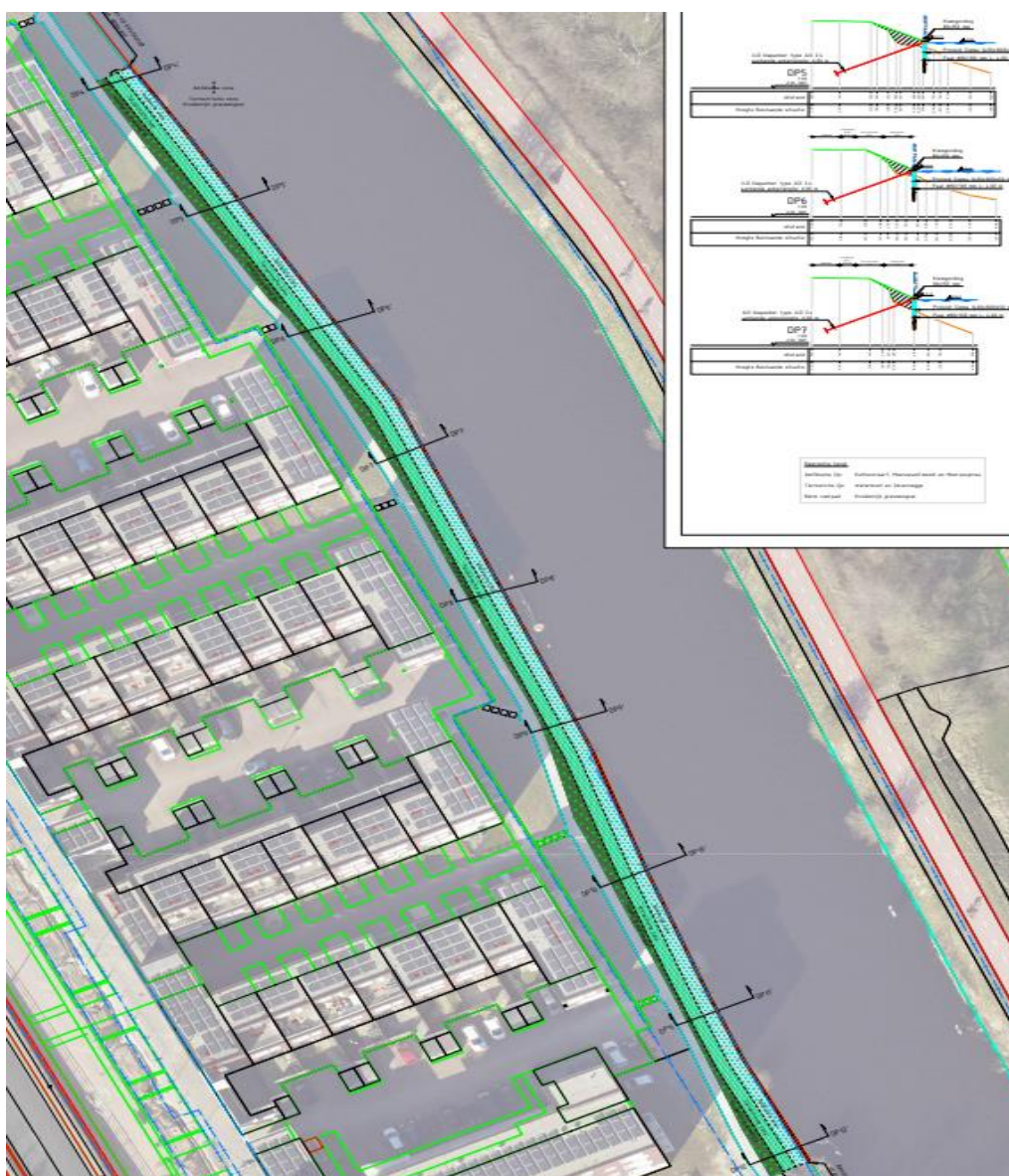
Figuur 1: Locatie te vervangen damwand.
