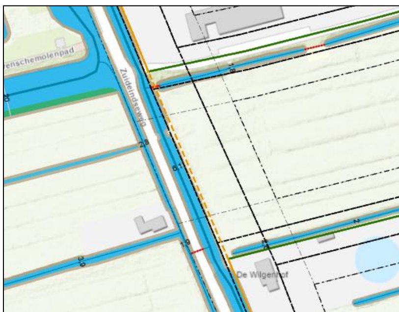
Figuur 3: Regionale kering Zuideindseweg 76 Delfgauw (gestreepte lijn geeft de doorgetrokken buitenkruinlijn van de waterkering weer).
