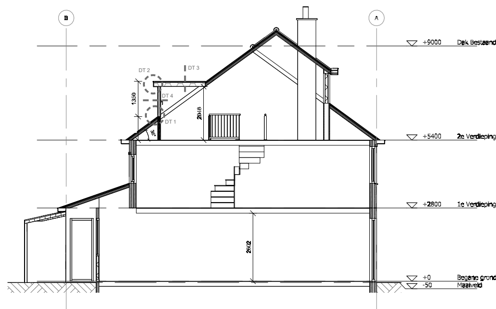
Doorsnede A-A (Nieuwe situatie) Schaal 1 : 100
