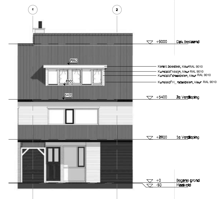
Voorgevel (Nieuwe situatie) Schaal 1 : 100
