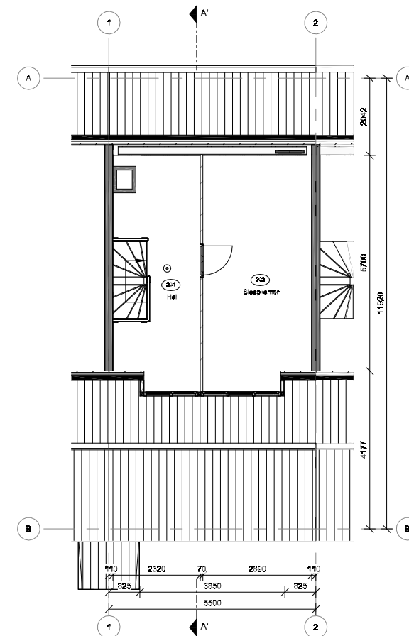
Tweede verdieping (Nieuwe situatie) Schaal 1 : 100
