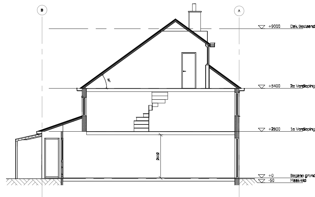
Doorsnede A-A (Bestaande situatie) Schaal 1 : 100
