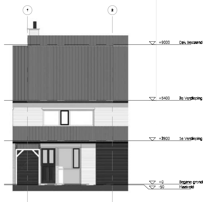
Voorgevel (Bestaande situatie) Schaal 1 : 100
