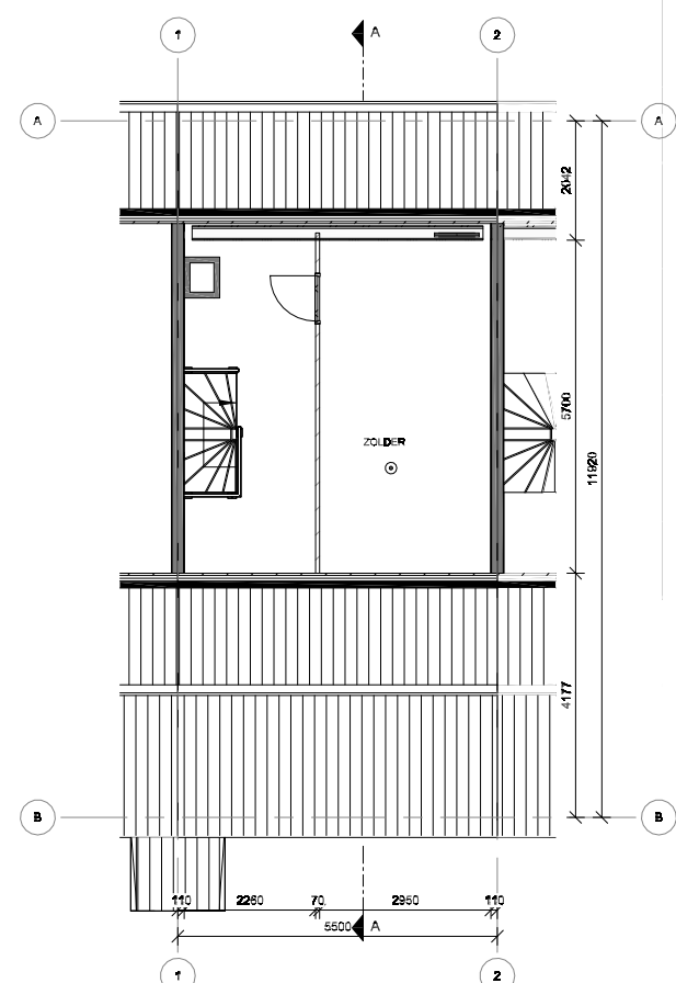
Tweede verdieping (Bestaande situatie) Schaal 1 : 100
