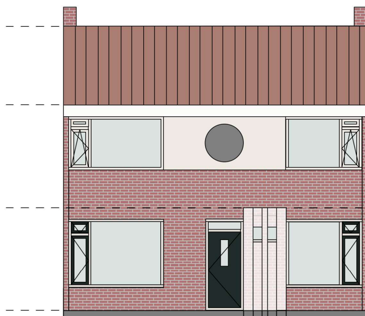
voorgevel
