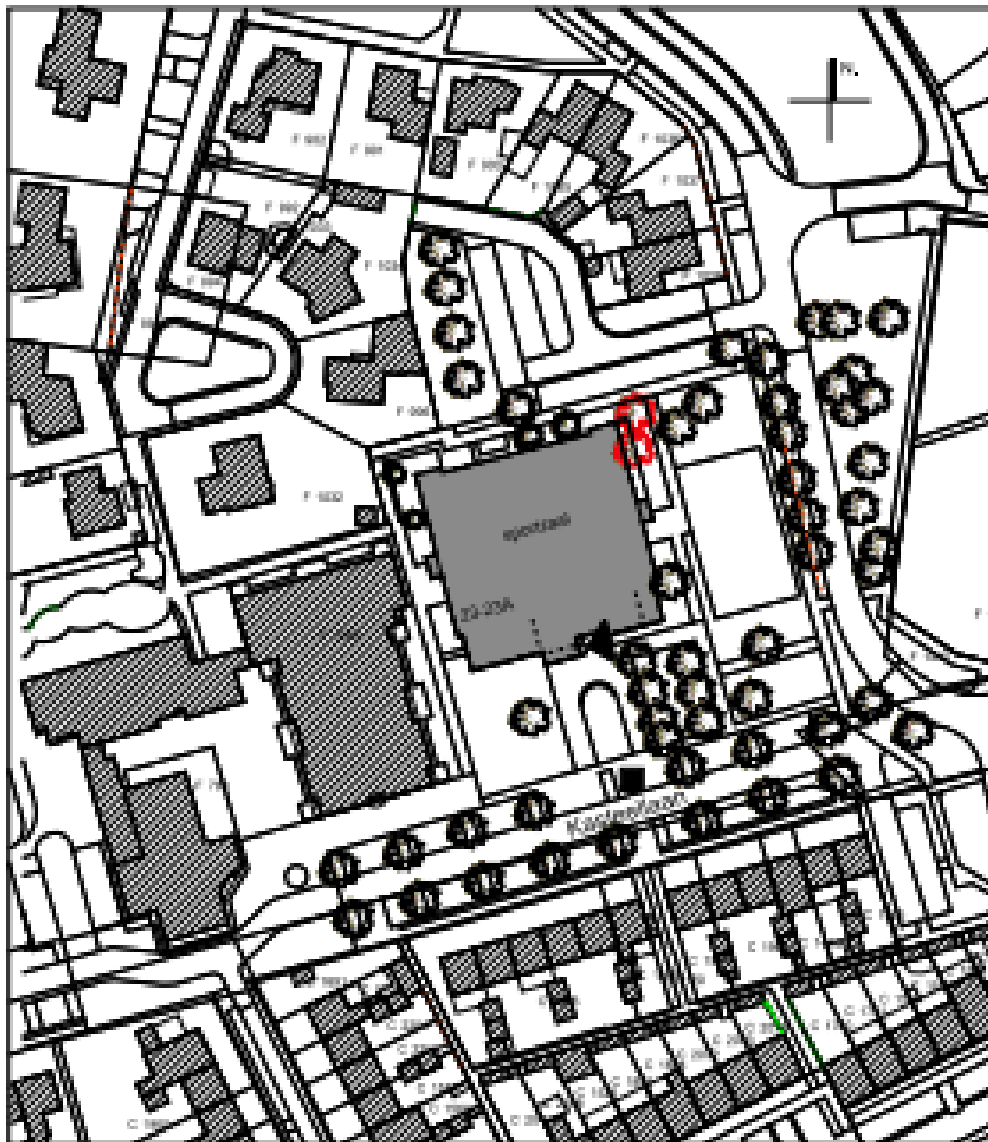
situatie schaal 1:1000
