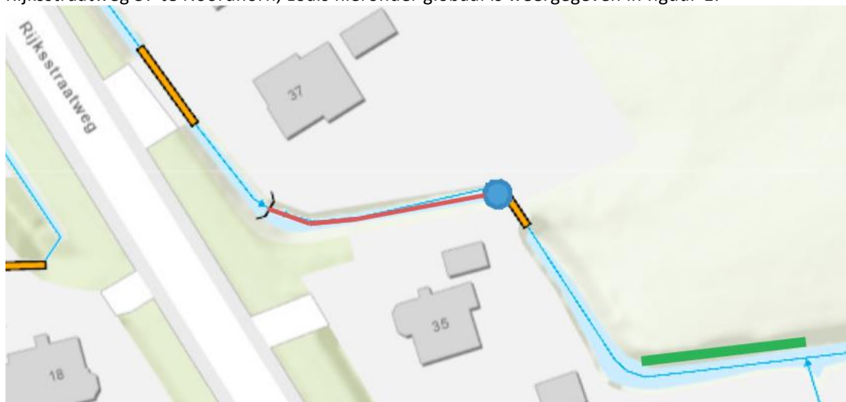
Figuur 1: Te dempen gedeelte weergegeven met rode lijn, te plaatsen inspectieput weergegeven met blauwe cirkel en gedeelte te verbreden watergang weergegeven met groene lijn.
