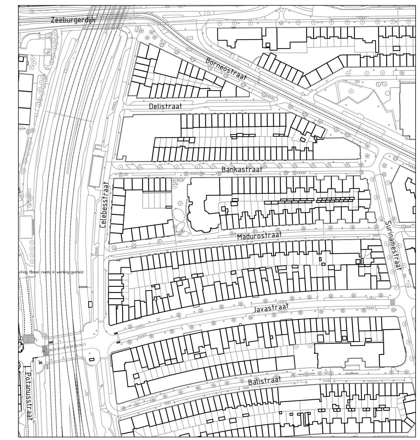
Situatie Javastraat Schaal 1:2000
