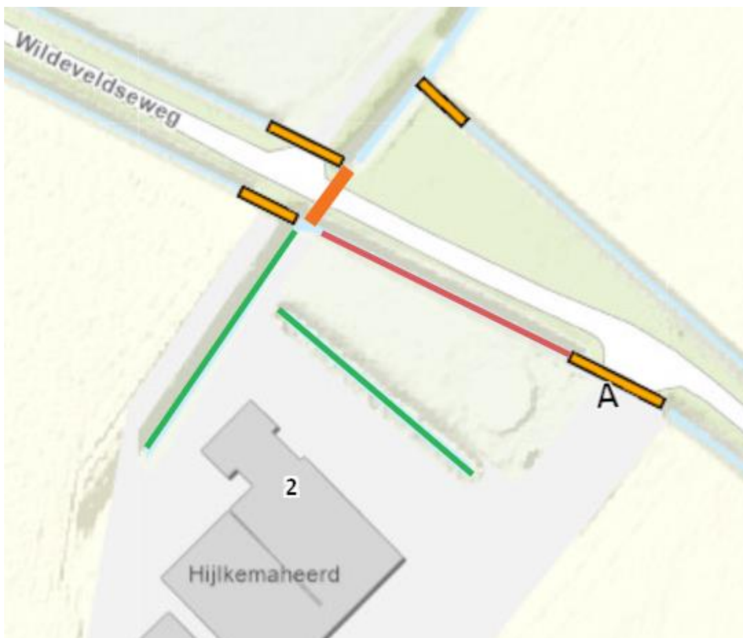
Figuur 1: Bestaande duikers weergegeven met oranje lijnen, te verlengen inritduiker weergegeven met 'A', slootdemping weergegeven met rode lijn, te verbreden watergangen weergegeven met groene lijnen.
