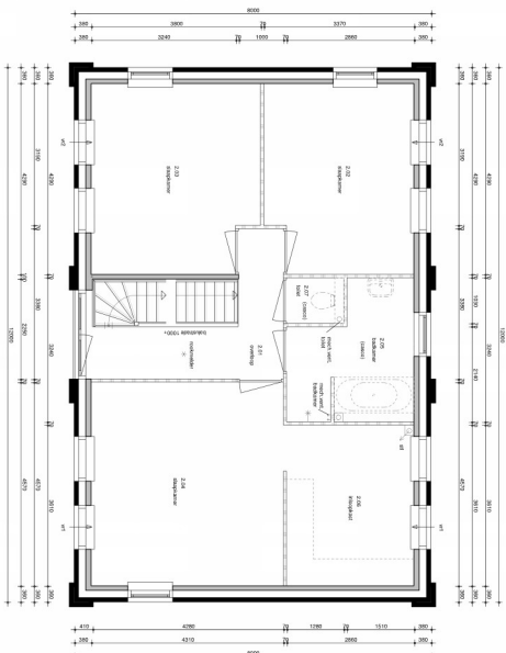
eerste verdieping 1 : 50
