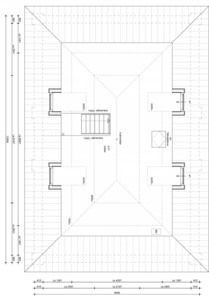
tweede verdieping 1 : 50
