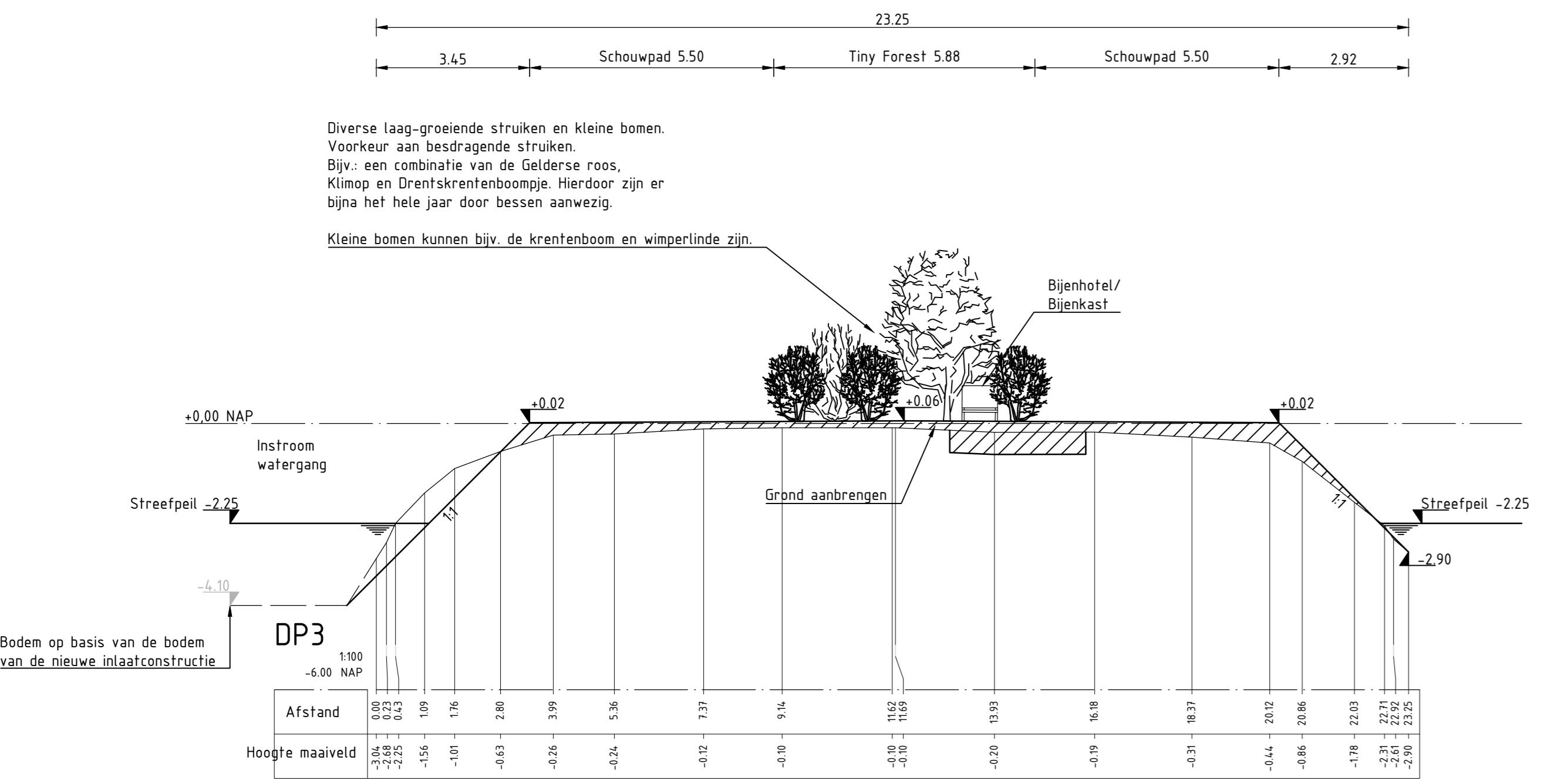
DWARSDOORSNEDE 3 SCHAAL 1 : 100
