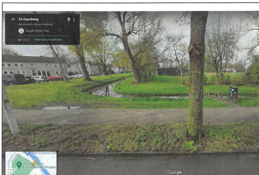
NOOIJ09.2 Situatie rondom de duiker, kijken vanaf de weg (Appelweg) richting sportpark Tuindorp Oostzaan en de bedieningskast van de meetinstrumenten.
