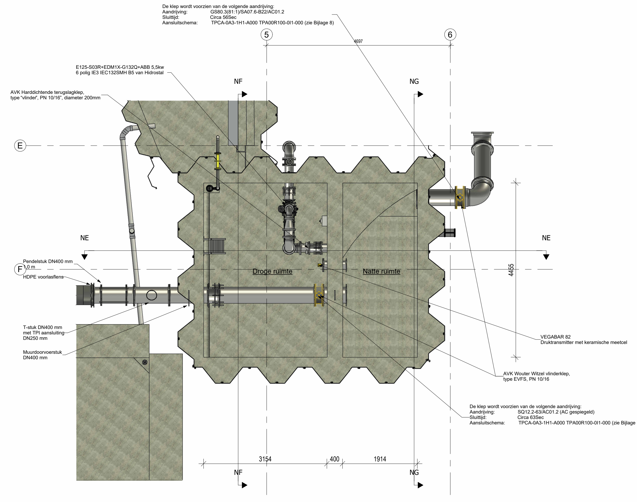
003 Visput -1.00 NAP
