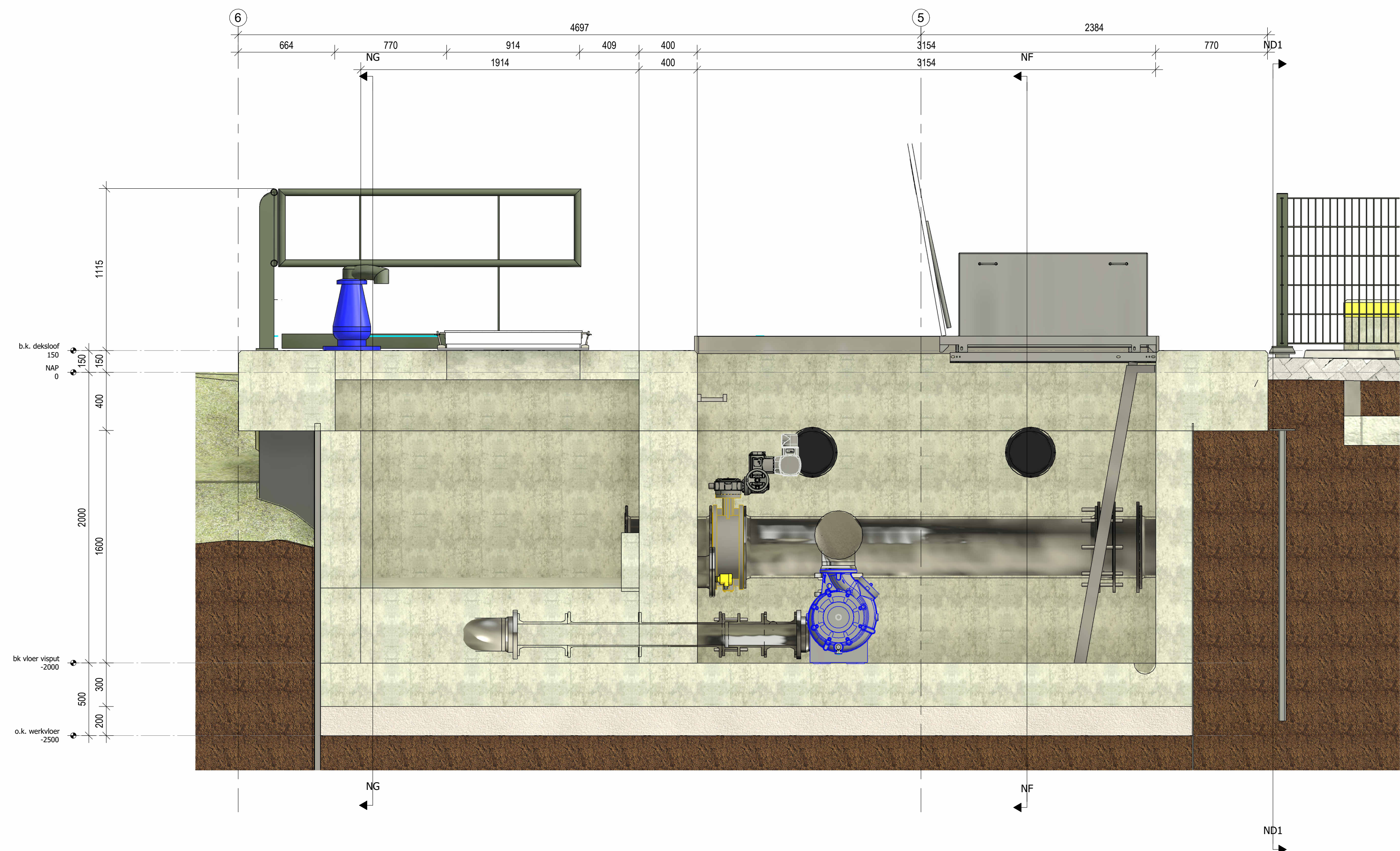
Doorsnede E-E
