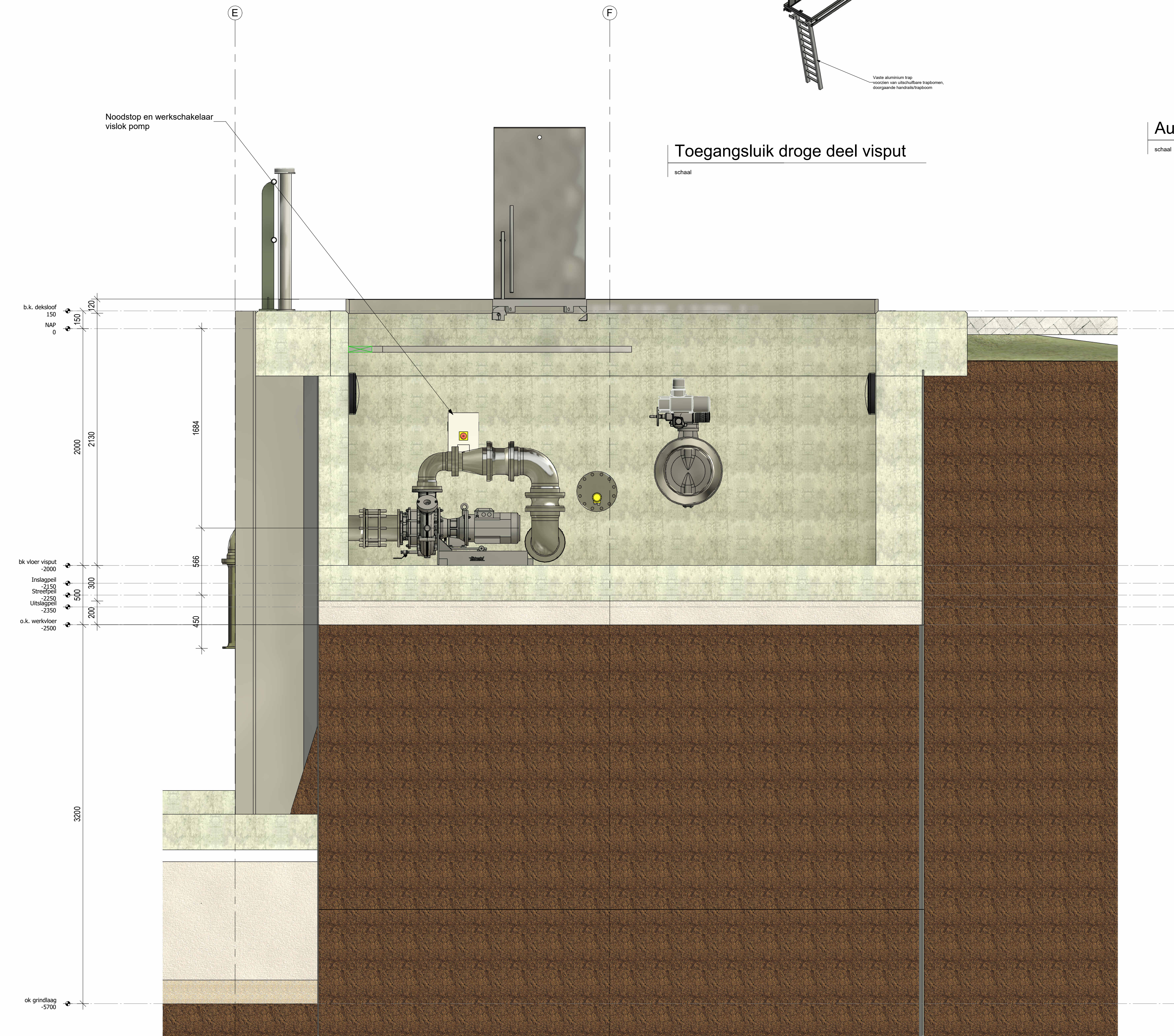
Doorsnede F-F
