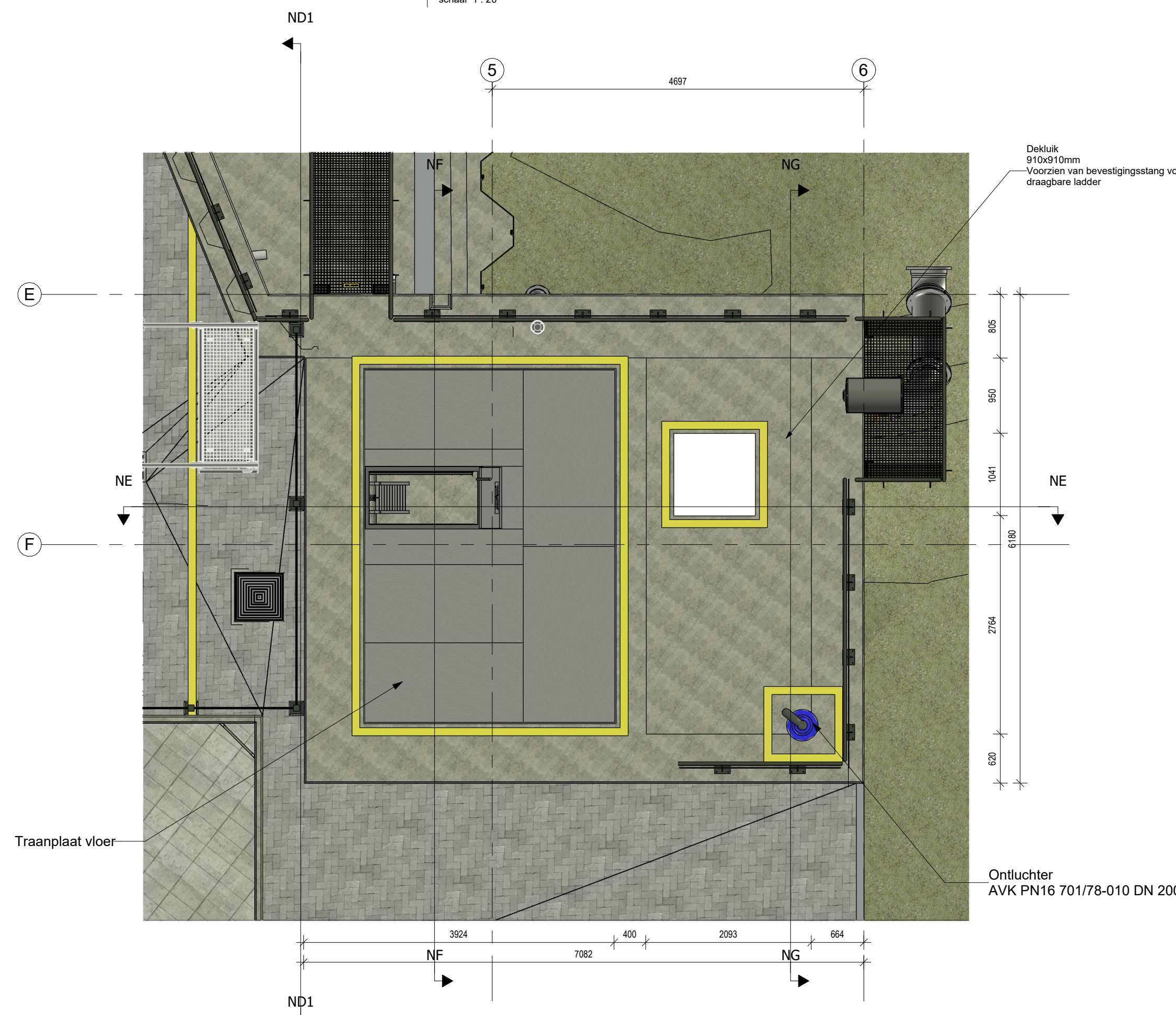
003 Visput +0.50 NAP
