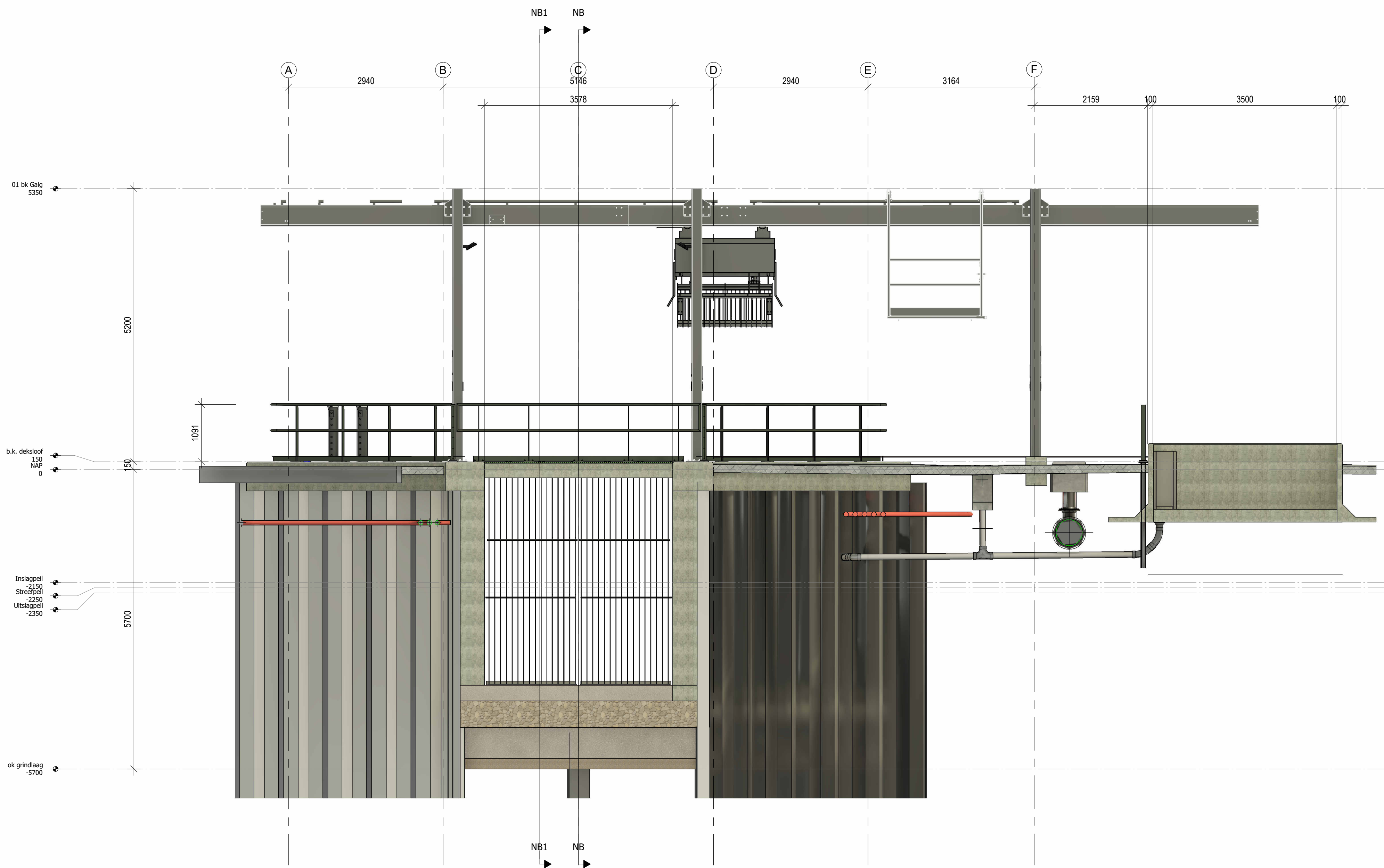
Doorsnede D-D
