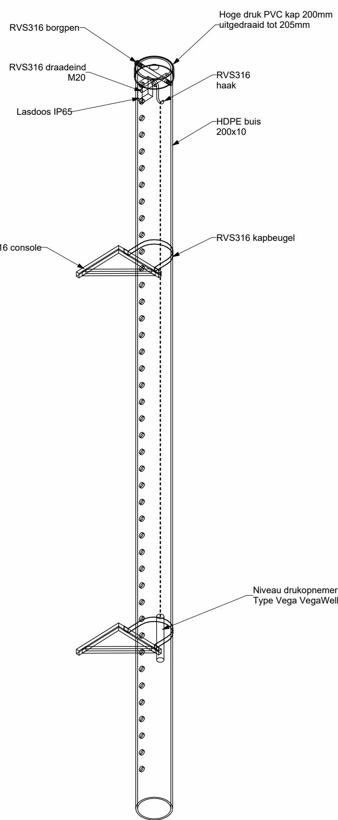
Peilbuis
