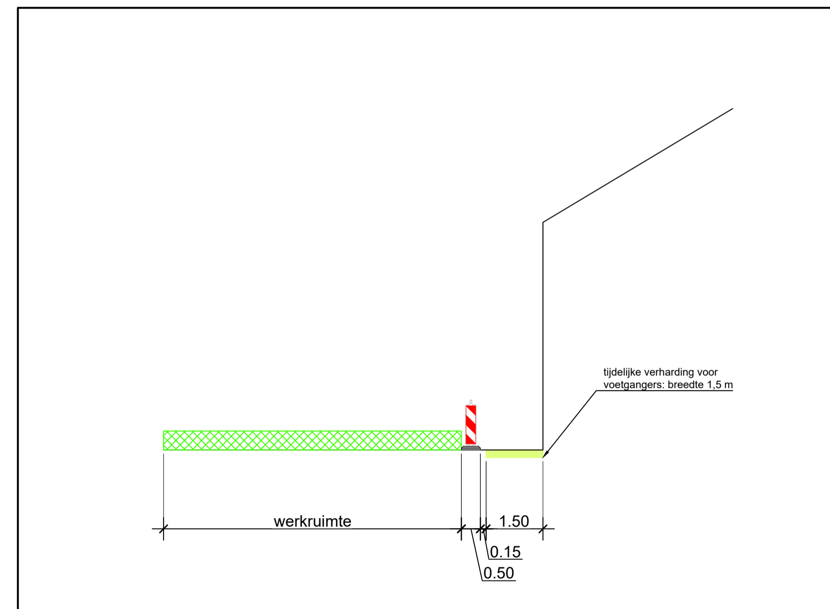
DOORSNEDEN A principe voetgangers door werkvak SCHAAL 1:100
