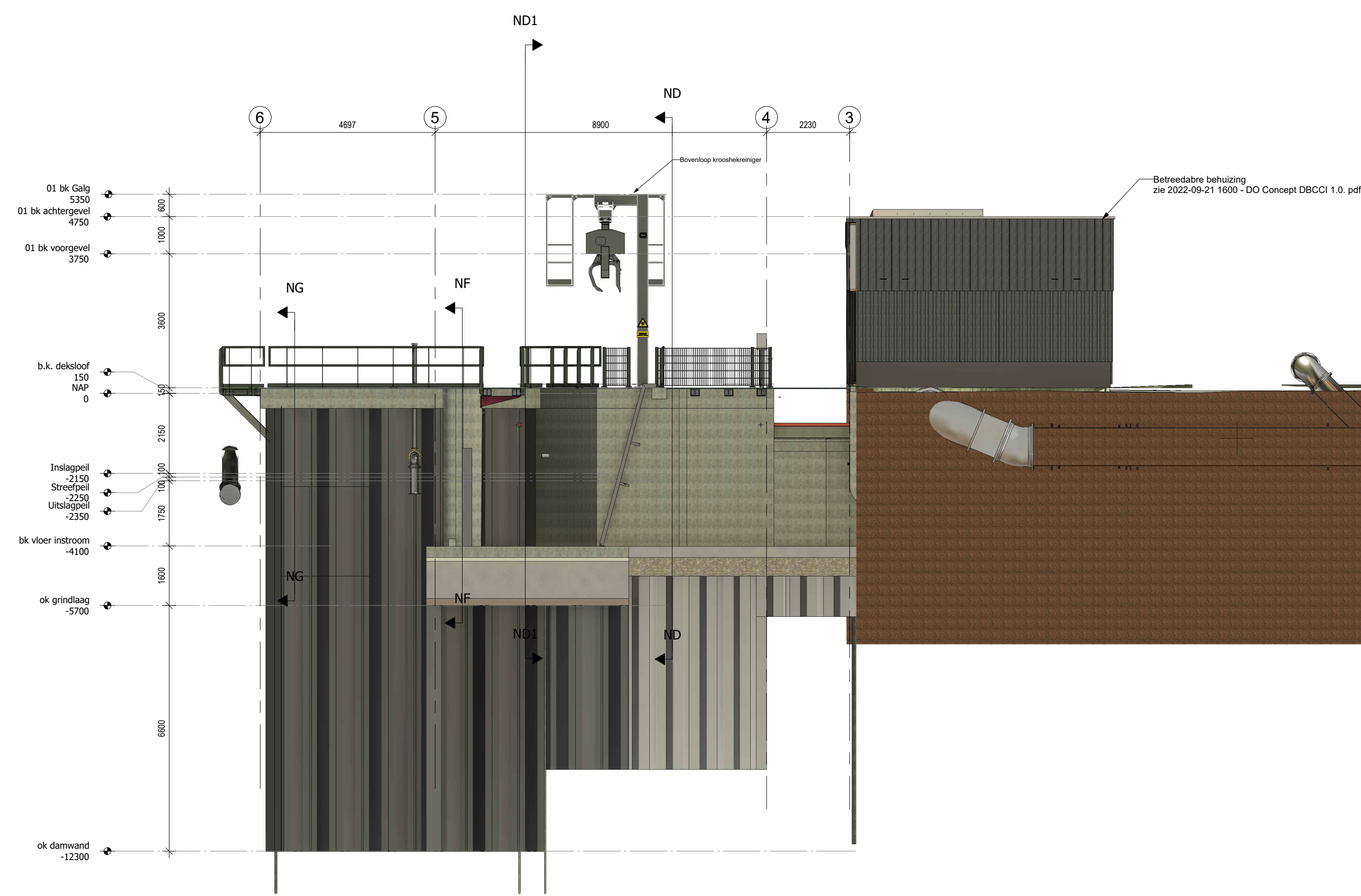
Doorsnede B1-B1
