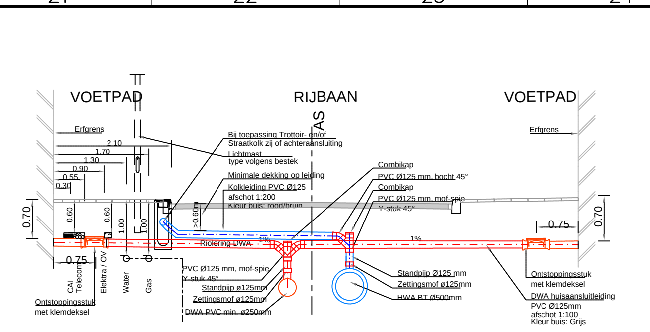
PRINCIPE DWARSPROFIEL A Kolk en fietsruimte met kabel en leidingtracé Schaal 1:50
