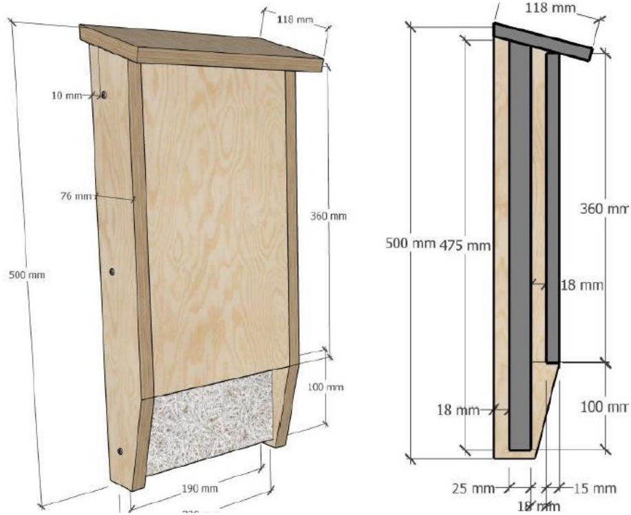
Afbeelding 3: Afmetingen van de platte tijdelijke vleermuiskasten.
