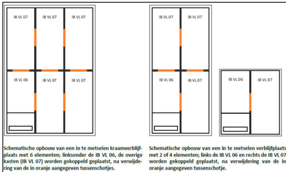
Afbeelding 6: Voorbeeld van de schematische opbouw van de in te metselen geschakelde vleermuiskasten (links: een kraamverblijfplaats (enkellaags), rechts: een paarverblijfplaats).
