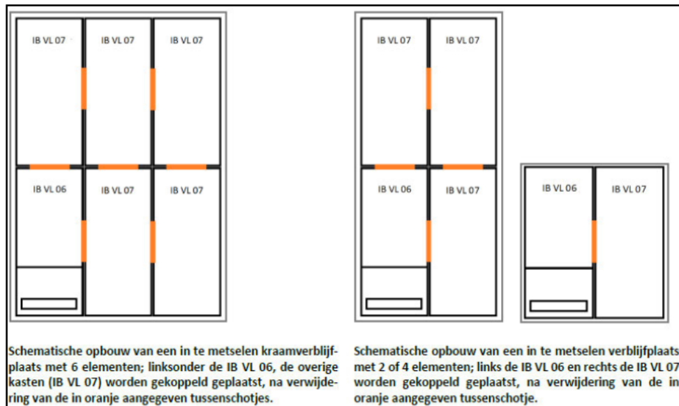
Afbeelding 7: Voorbeeld van de schematische opbouw van de in te metselen geschakelde vleermuiskasten (links: een kraamverblijfplaats (mogelijke invulling, enkellaags), rechts: een zomer- en/of paarverblijfplaats).
