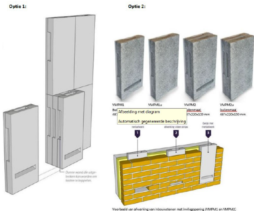
Afbeelding 8: Voorbeeld van de schematische opbouw van de in te metselen geschakelde vleermuiskasten voor de kraamverblijfplaats (mogelijke invulling, dubbellaags).
