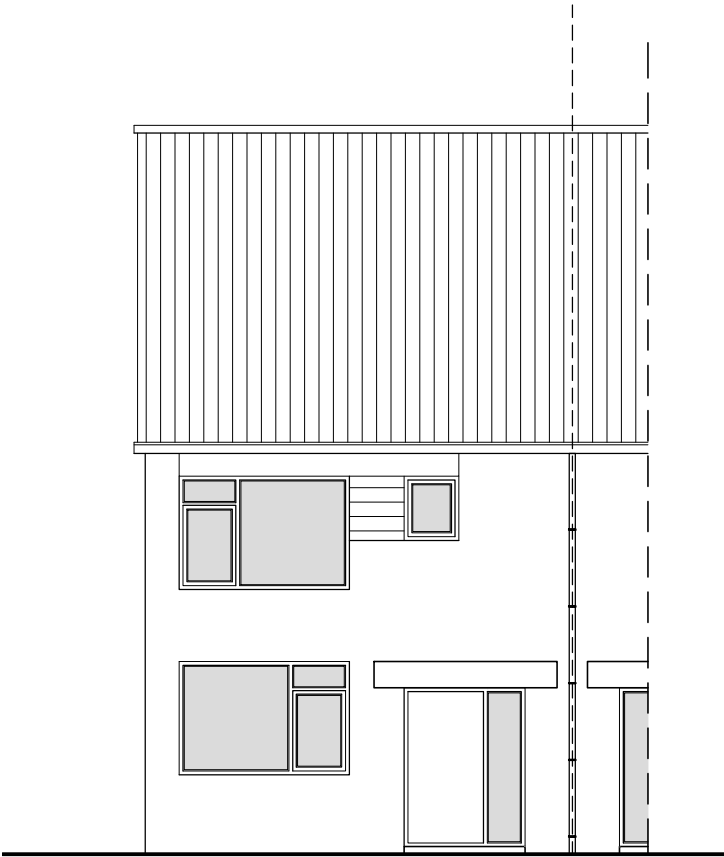
Voorgevel (Bestaande situatie)
