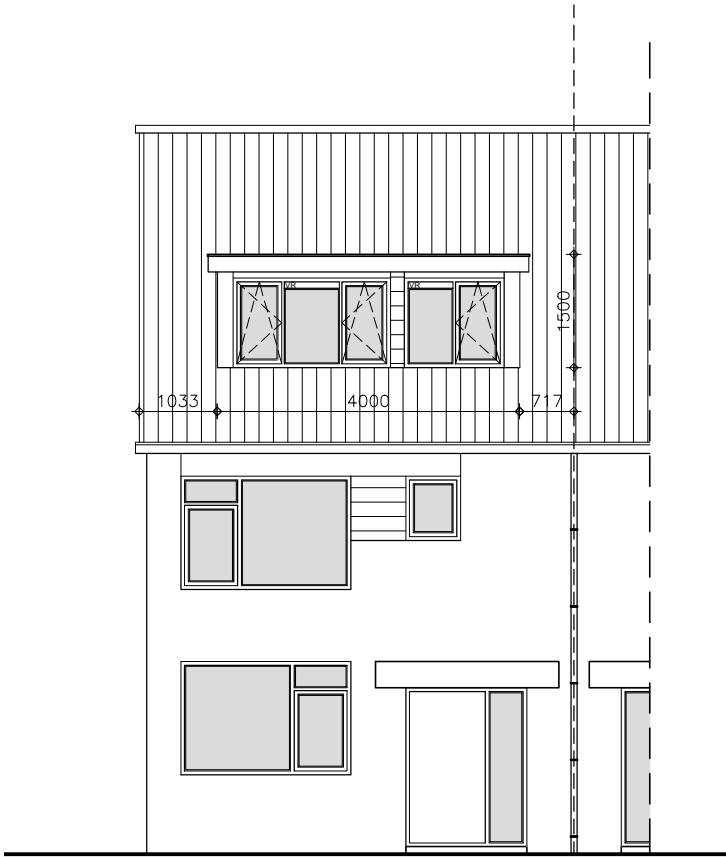
Voorgevel (Nieuwe situatie)
