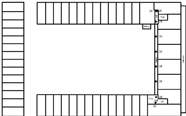
2e Verdieping
