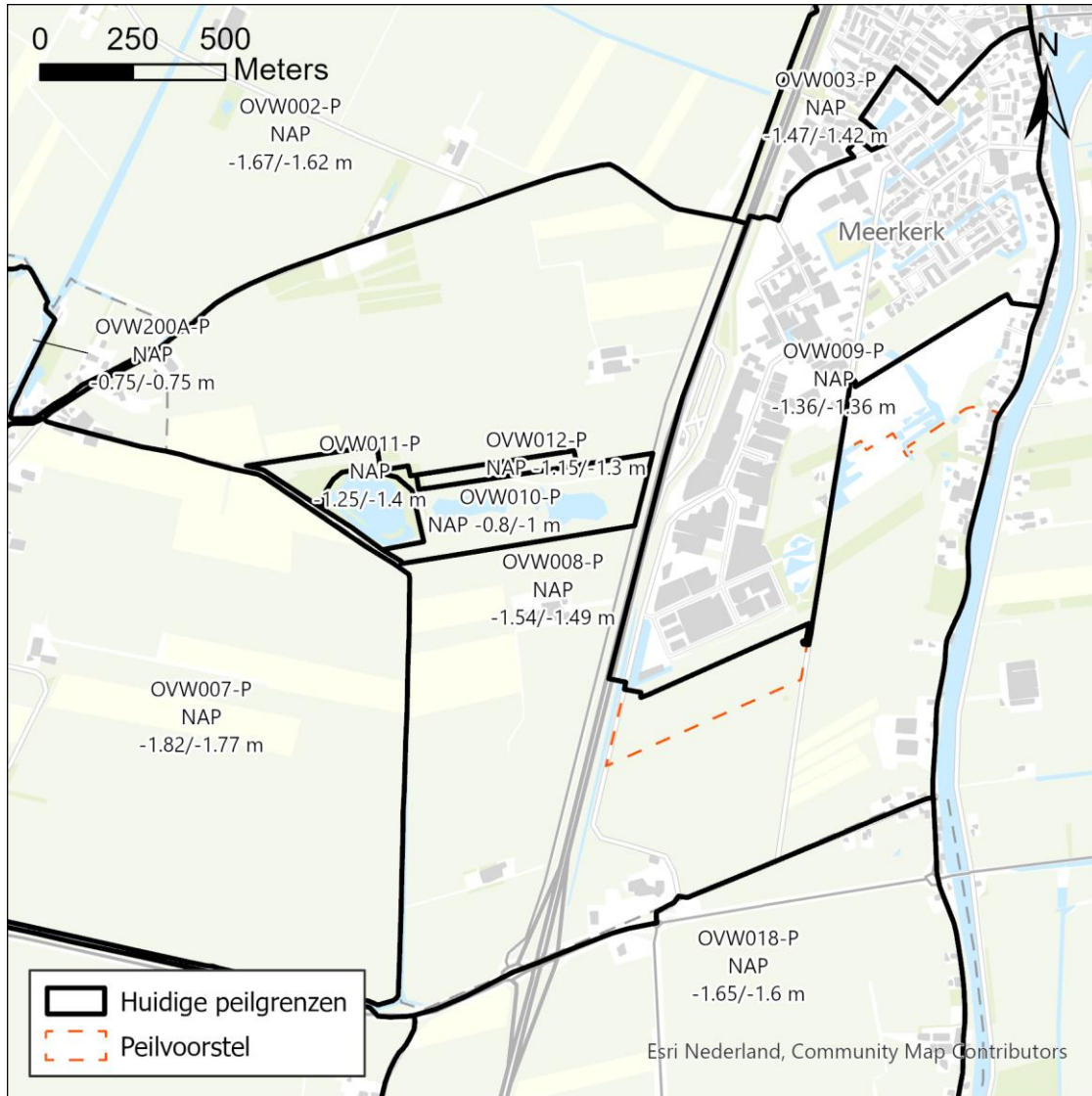
Afbeelding IX.1 Peilmaatregel OVW008/OVW009
