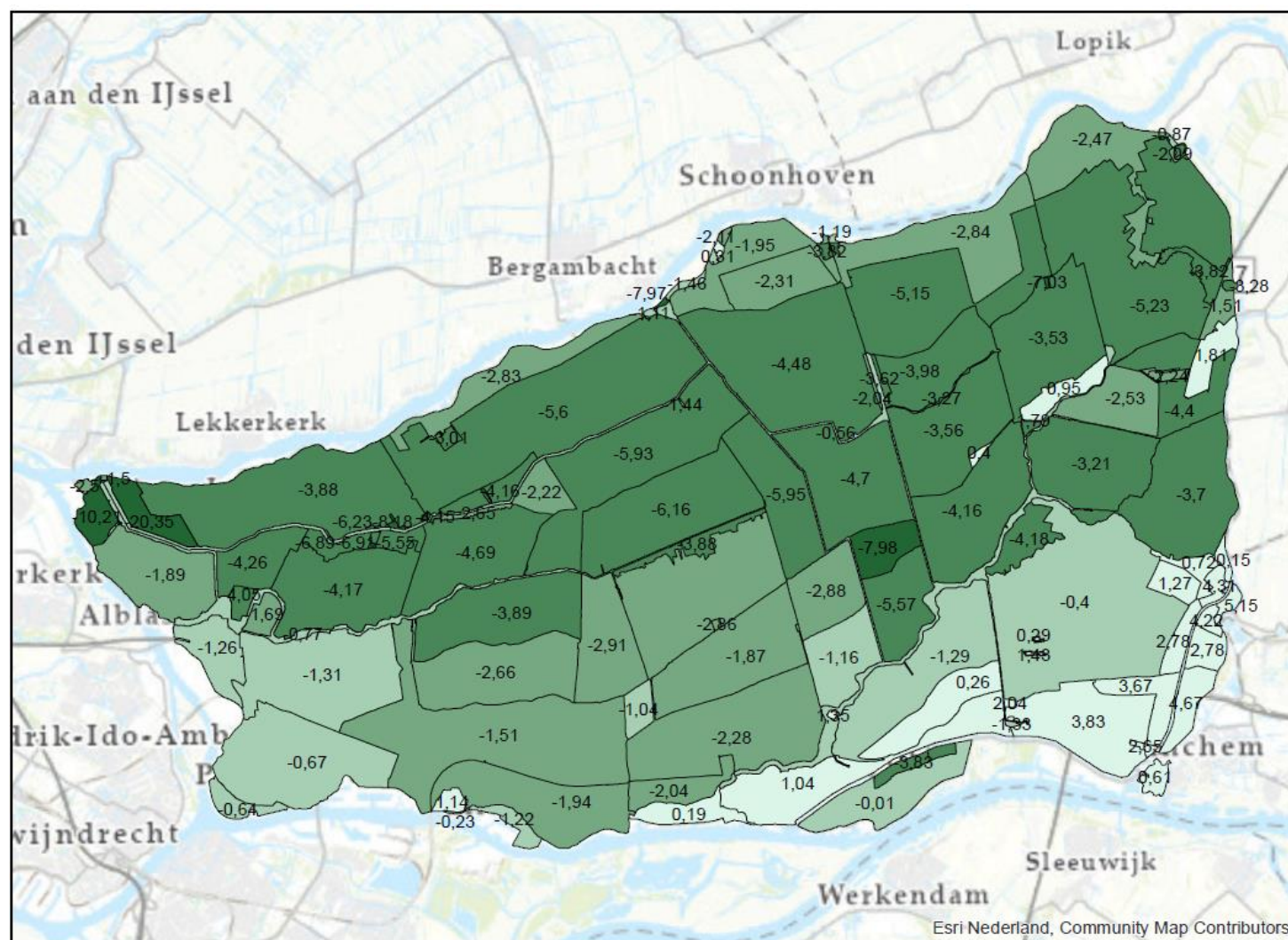
Kaart 11: Bodemdalingskaart
