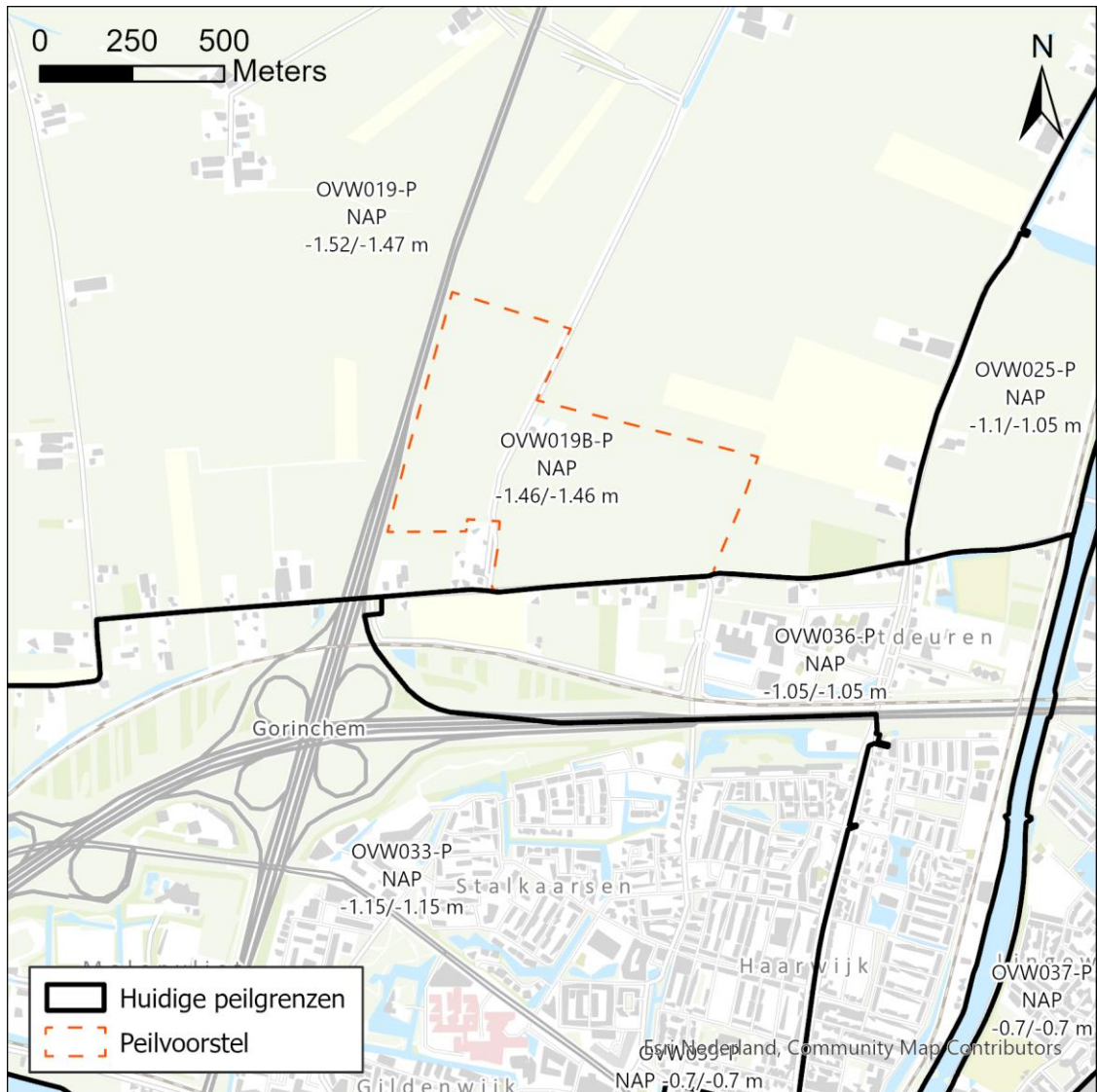
Afbeelding IX.1 Peilmaatregel OVW019B
