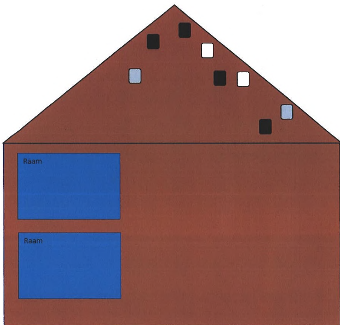
Figuur 10 | Voorstel voor plaatsing van tijdelijke vleermuiskasten (witte vierkanten: witte vleermuiskasten, zwarte vierkanten: zwarte vleermuiskasten en grijze vierkanten: grijze vleermuiskasten) (Thorbeckestraat 28)
