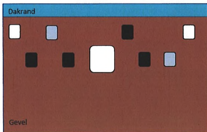
Figuur 16 | Voorstel voor plaatsing van tijdelijke vleermuiskasten (witte vierkanten: witte vleermuiskasten, zwarte vierkanten: zwarte vleermuiskasten en grijze vierkanten: grijze vleermuiskasten) (Plantsoenlaan 135)
