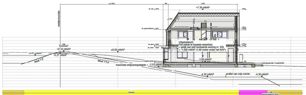
Fig. 5.4 Situering woning t.o.v. profielvrijeruimte
