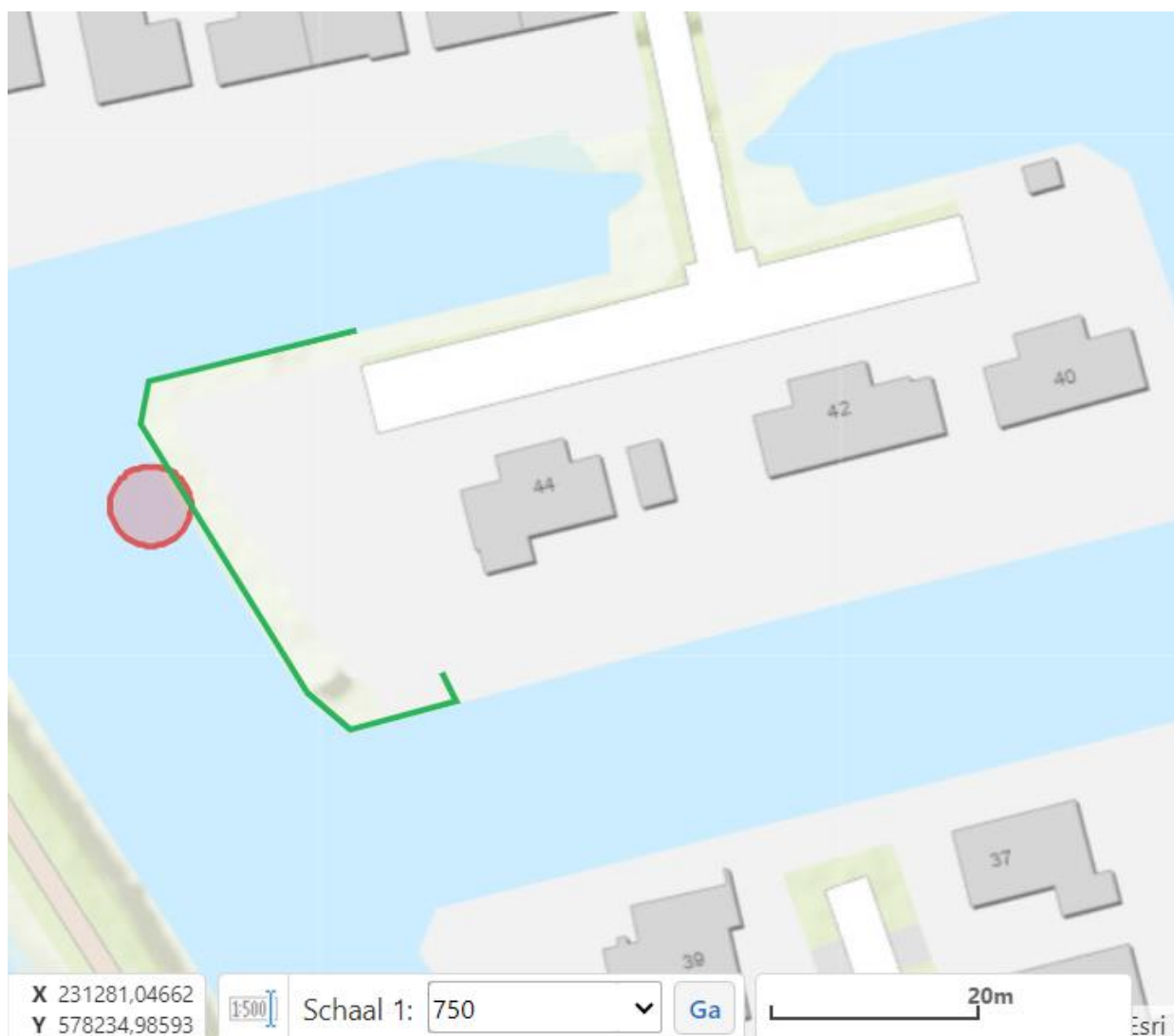
Figuur 1: Schematische tekening van de werkzaamheden. De rode cirkel geeft globaal de locatie weer van de aan te leggen steiger. De groene lijn geeft globaal de locatie weer van reeds aangelegde beschoeiing.
