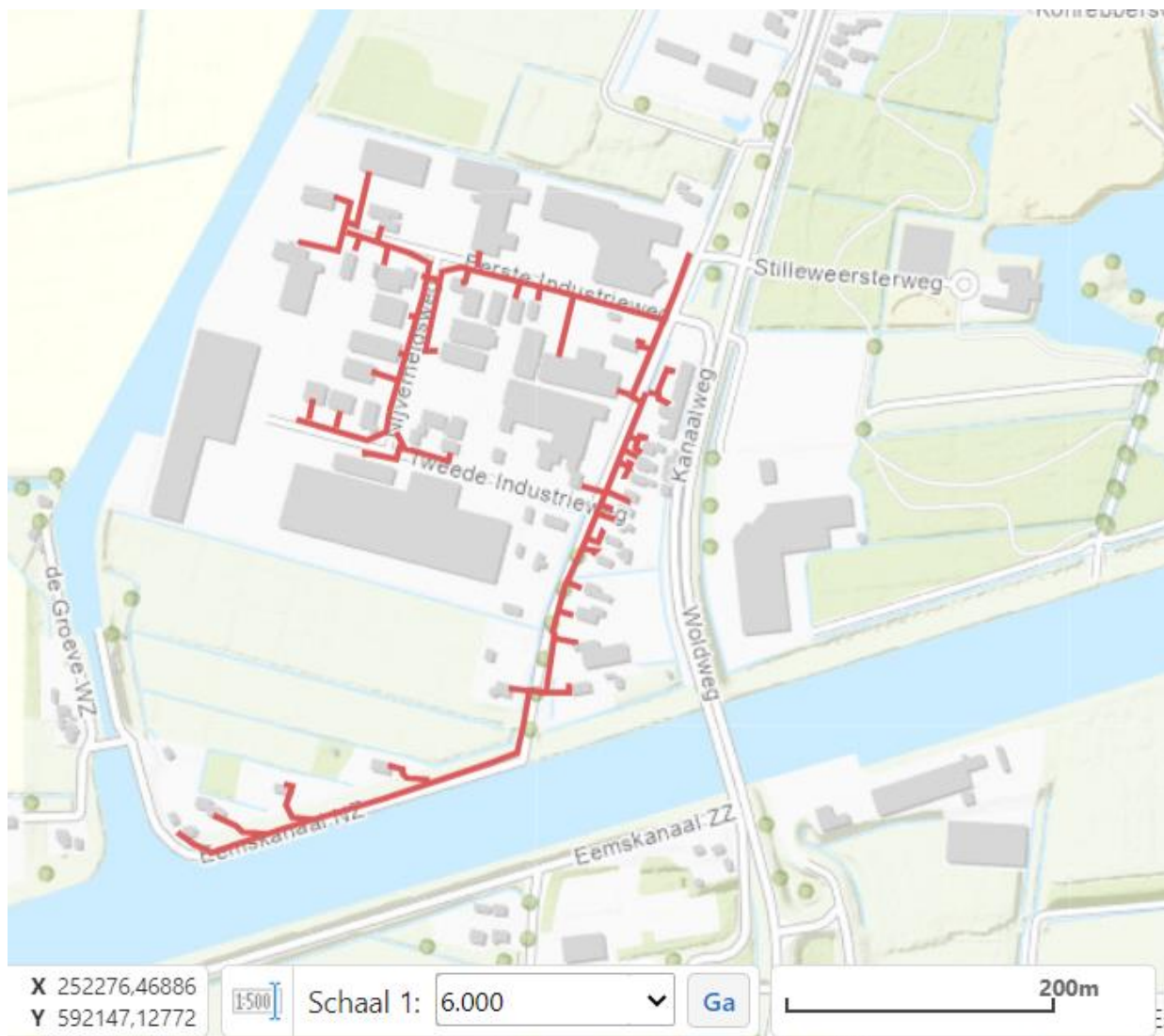
Figuur 1: Schematische tekening van de werkzaamheden. De rode lijn geeft globaal de locaties weer van het aan te leggen tracé.
