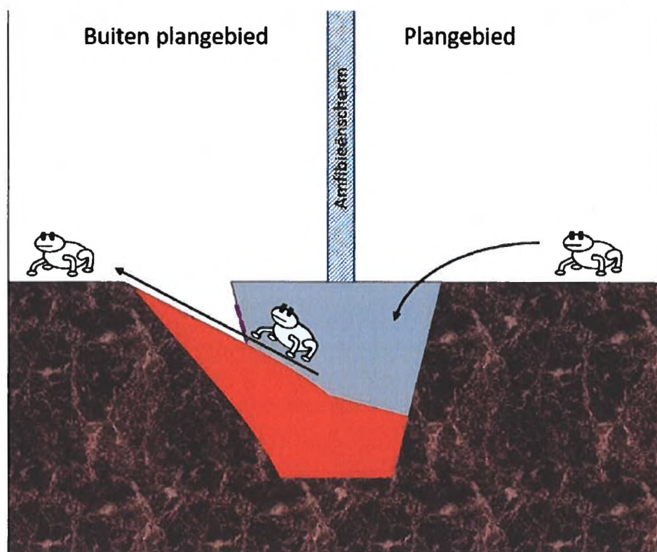
Figuur 4.2 Opstelling scherm en emmer die dieren de mogelijkheid geeft op eigen kracht een uitgerasterd terrein te verlaten. (H. Melchers Habitus)
