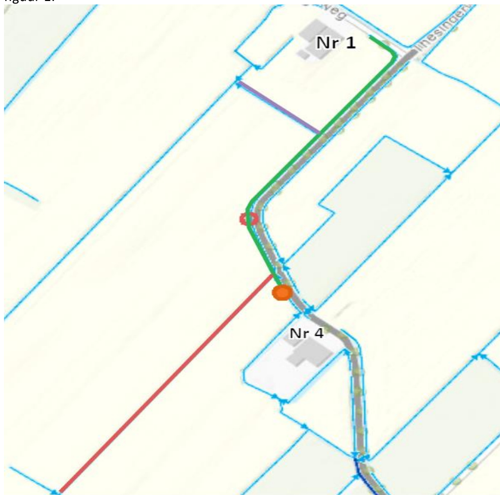
Figuur 1: Te verwijderen dam weergegeven met rode cirkel, te verbreden dam weergegeven met oranje cirkel, te dempen watergang weergegeven met rode lijn, reeds verbrede watergang weergegeven met paarse lijn en (nog) te verbreden watergang weergegeven met groene lijn.
