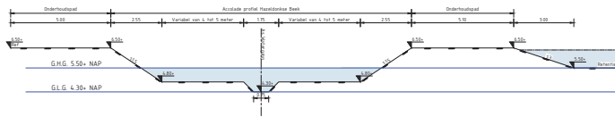
Principedoorsnede Hazeldonksebeek (Accoladeprofiel) 1:50
