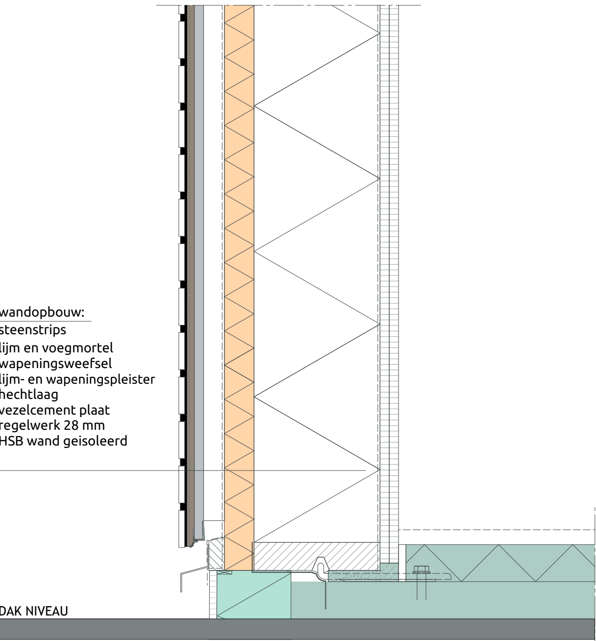
PRINCIPE DETAIL NIEUWE WAND
