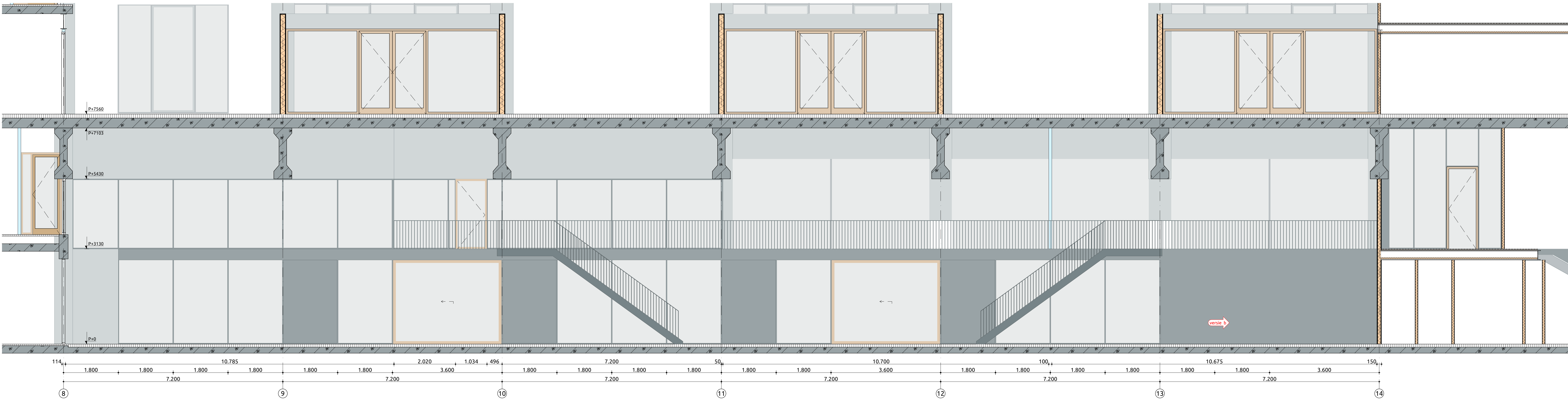
Binnengevel 04 1:50
