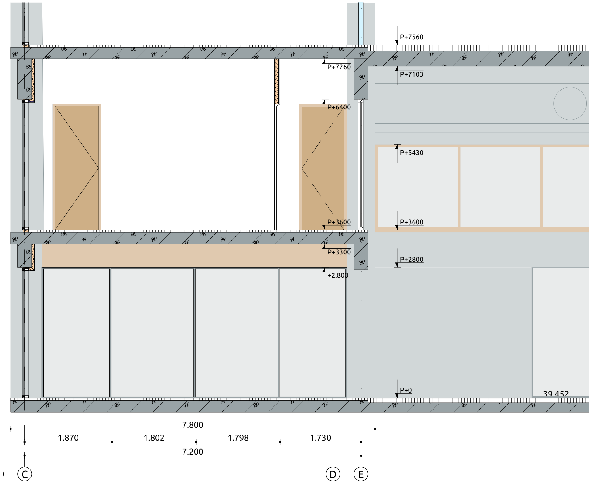
Binnengevel 02 1:50
