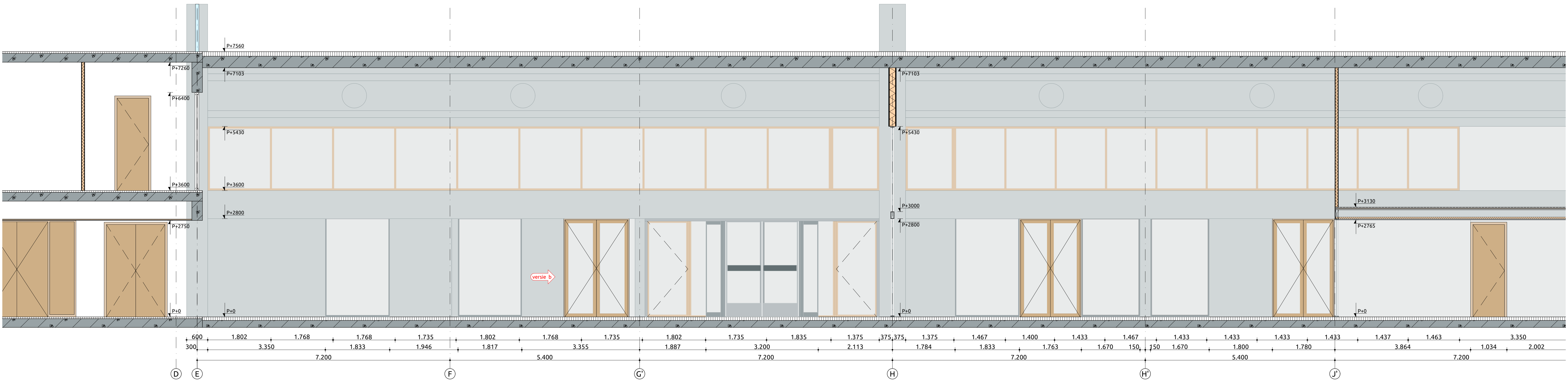
Binnengevel 05 1:50
