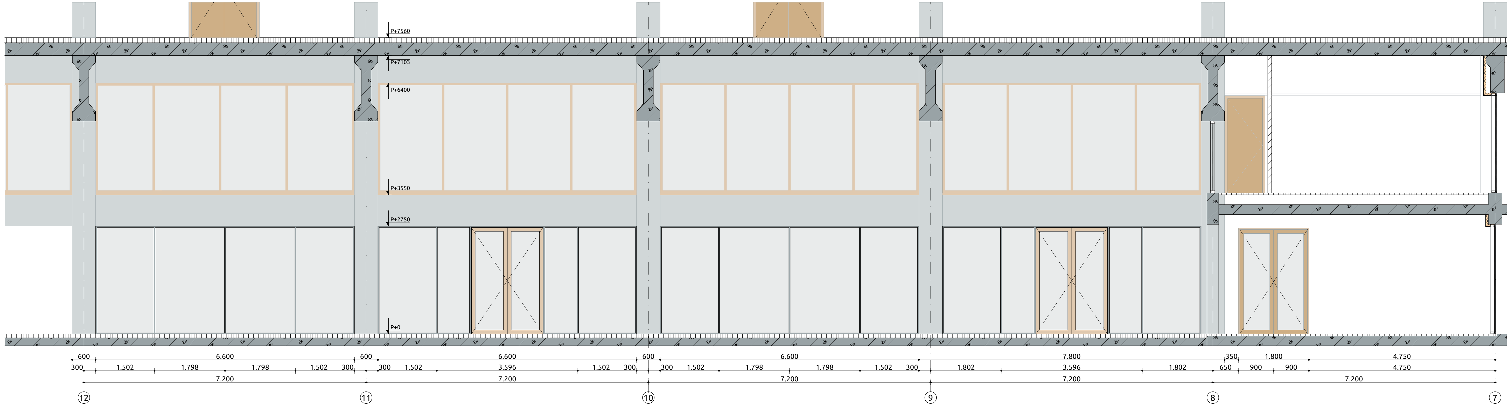
Binnengevel 03 1:50
