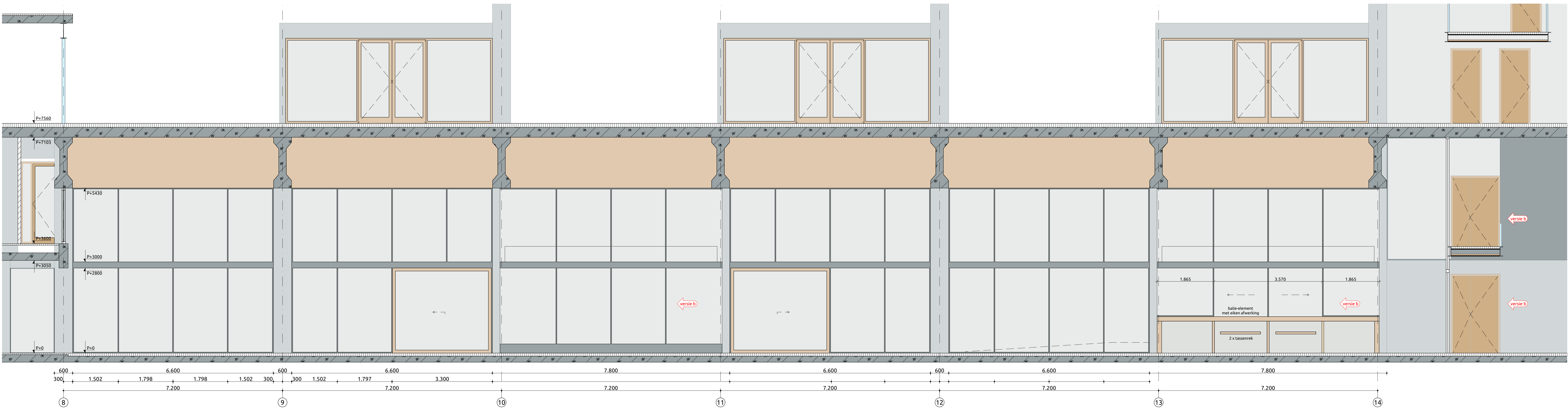
Binnengevel 01 1:50
