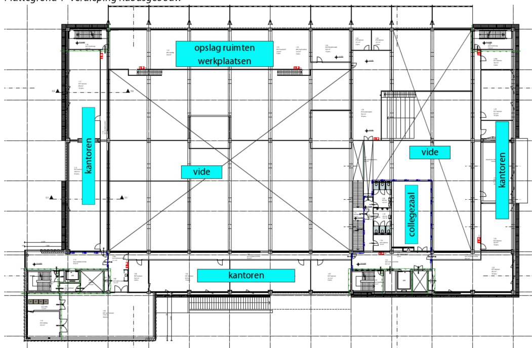
f2.3 Plattegrond 1 e verdieping Kubusgebouw
