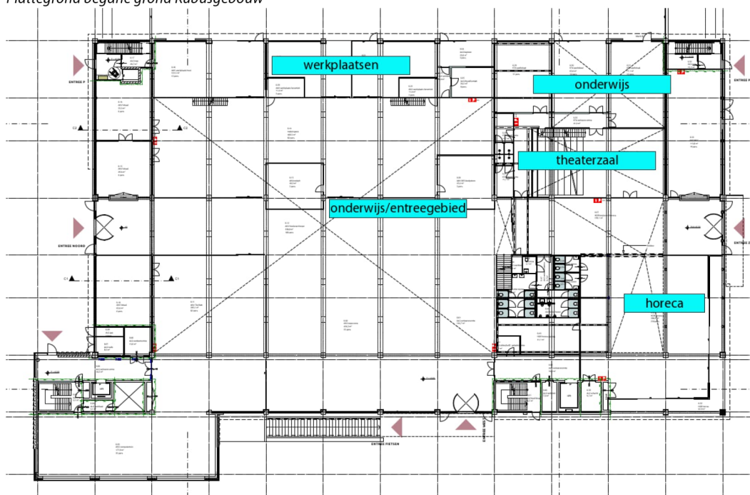
f2.2 Plattegrond begane grond Kubusgebouw
