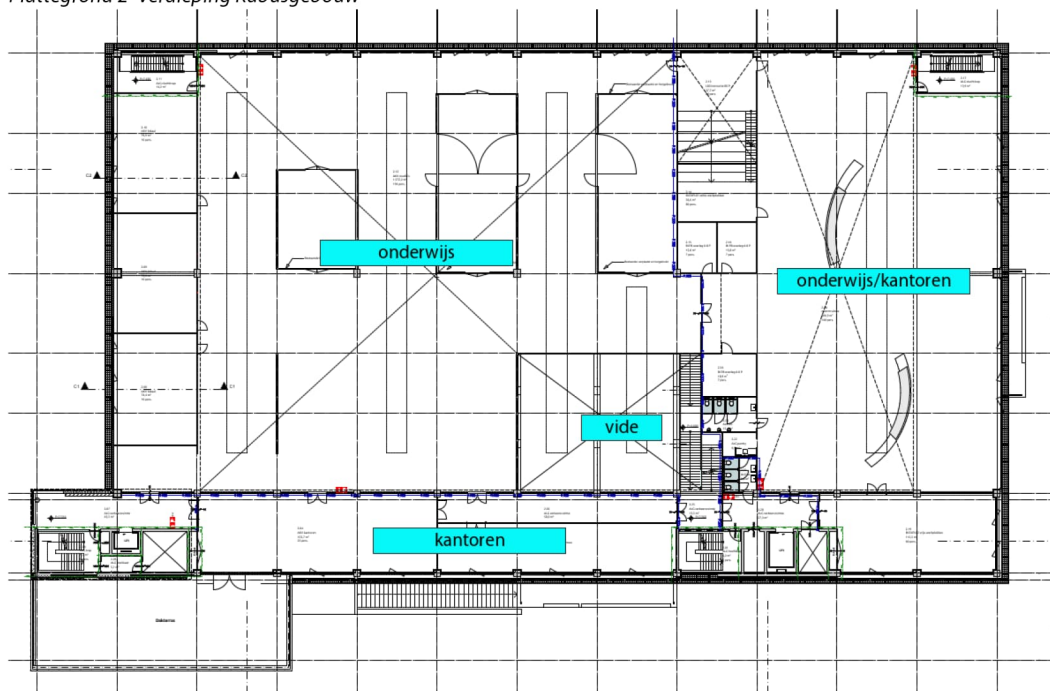
f2.4 Plattegrond 2 e verdieping Kubusgebouw
