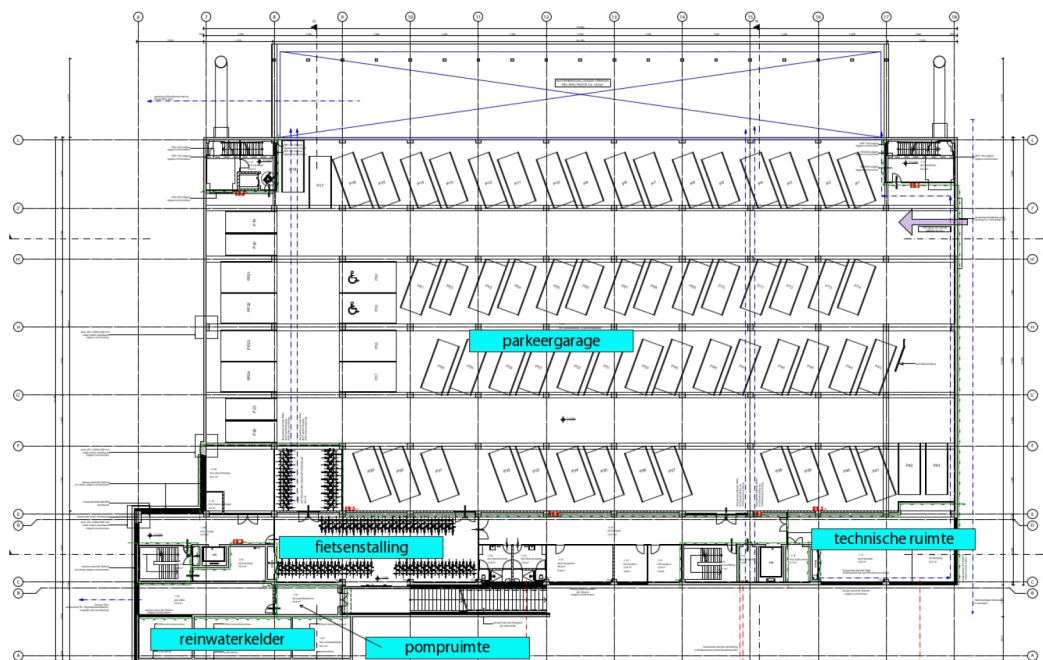
f2.1 Plattegrond kelder Kubusgebouw
