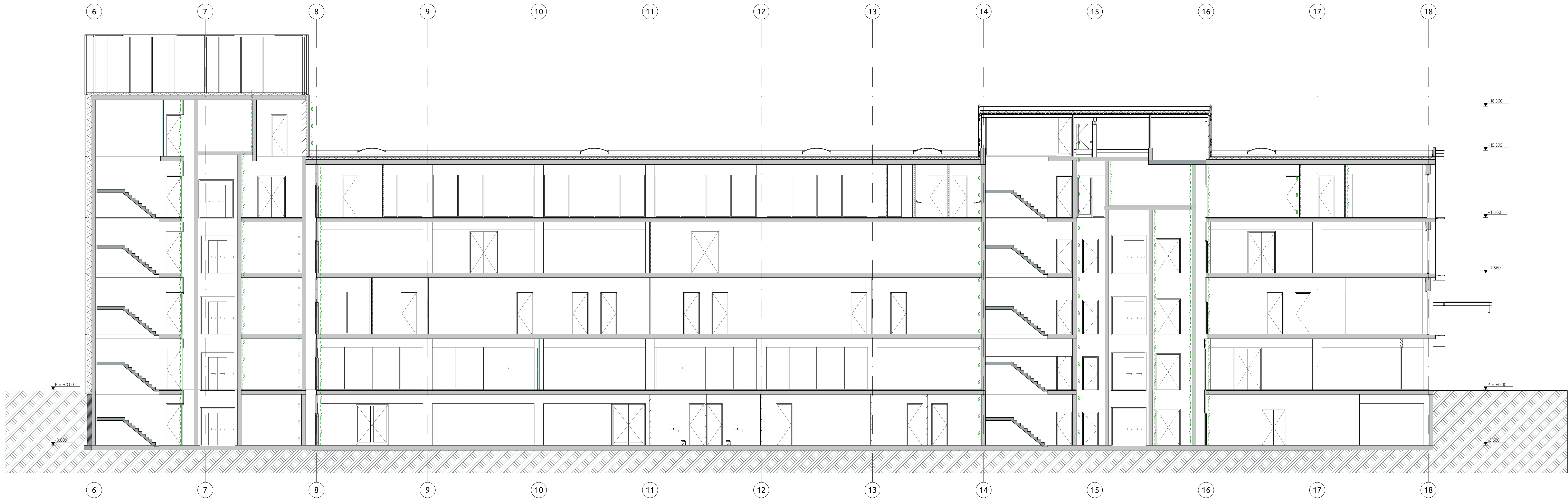
Doorsnede B-B
