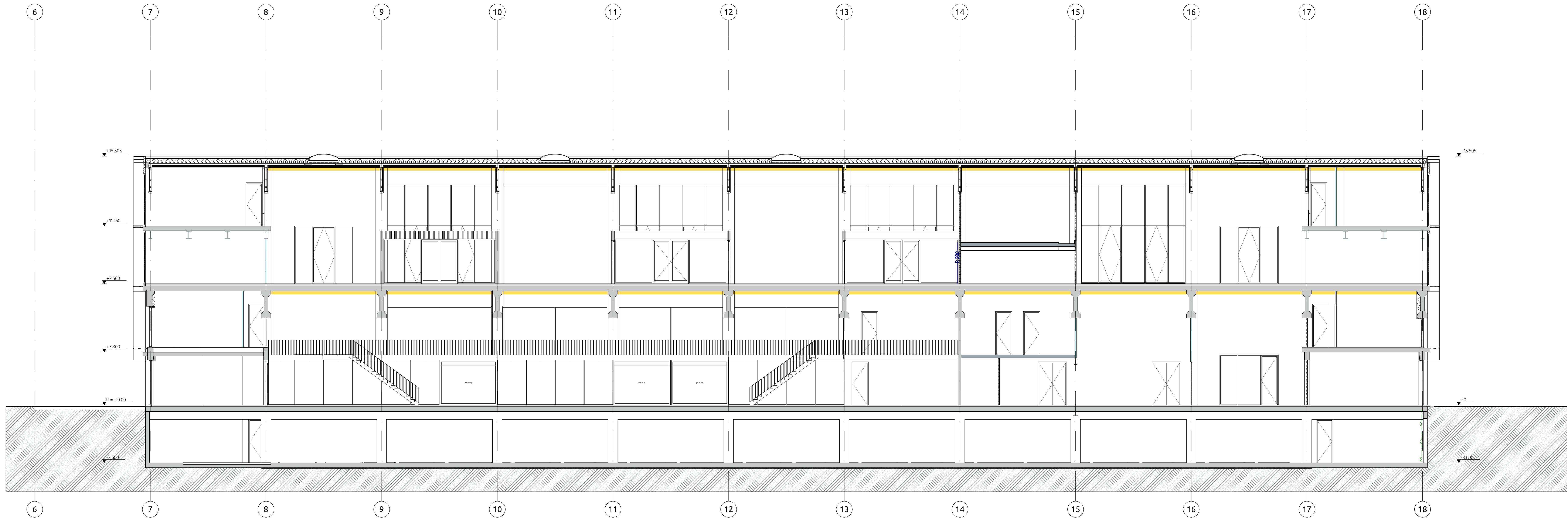
Doorsnede C-C
