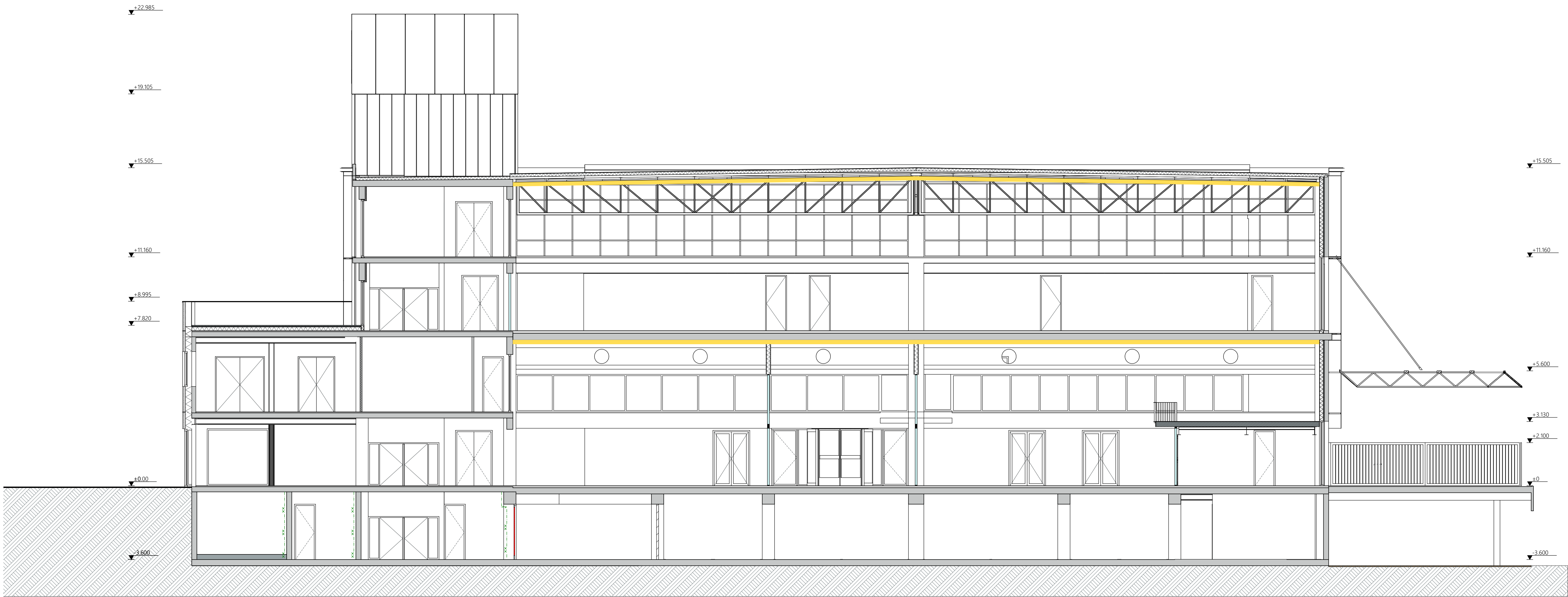
Doorsnede D-D
