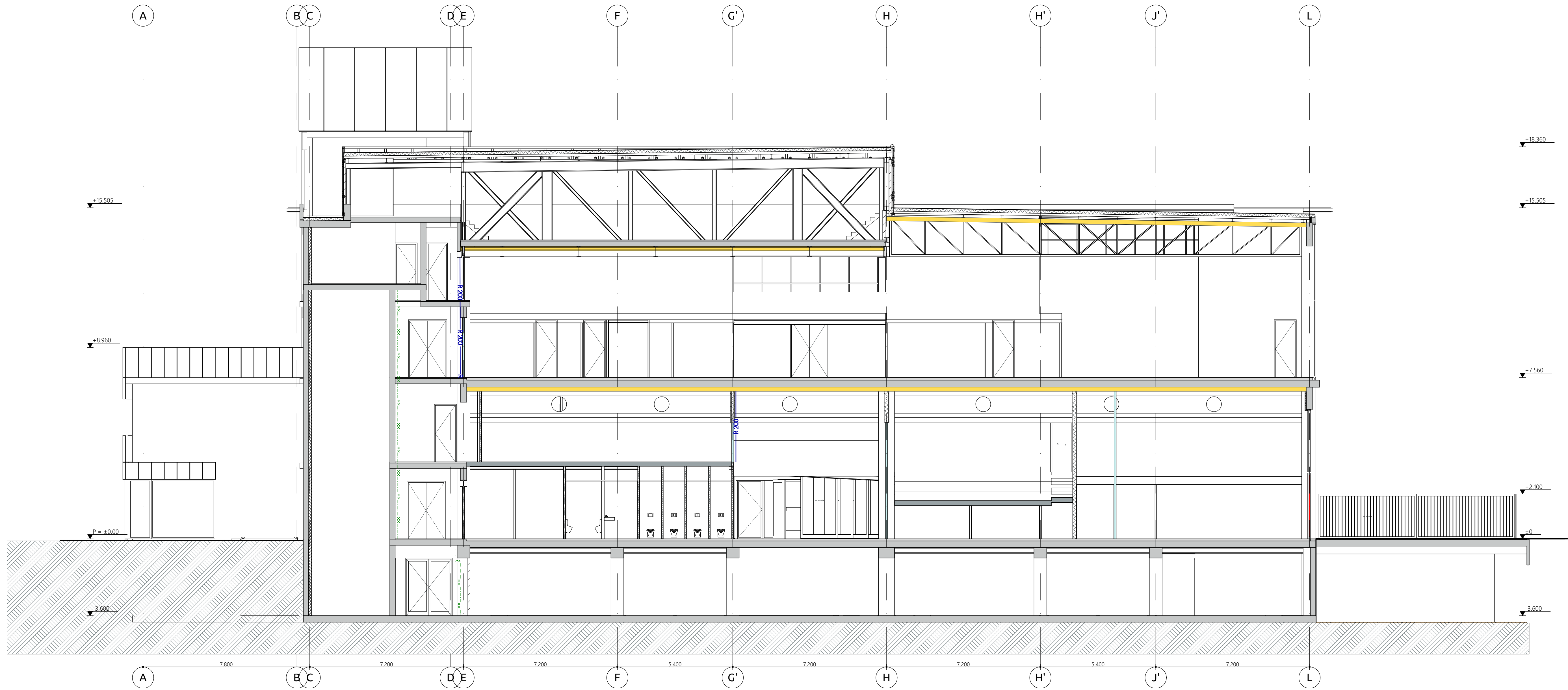
Doorsnede A-A
