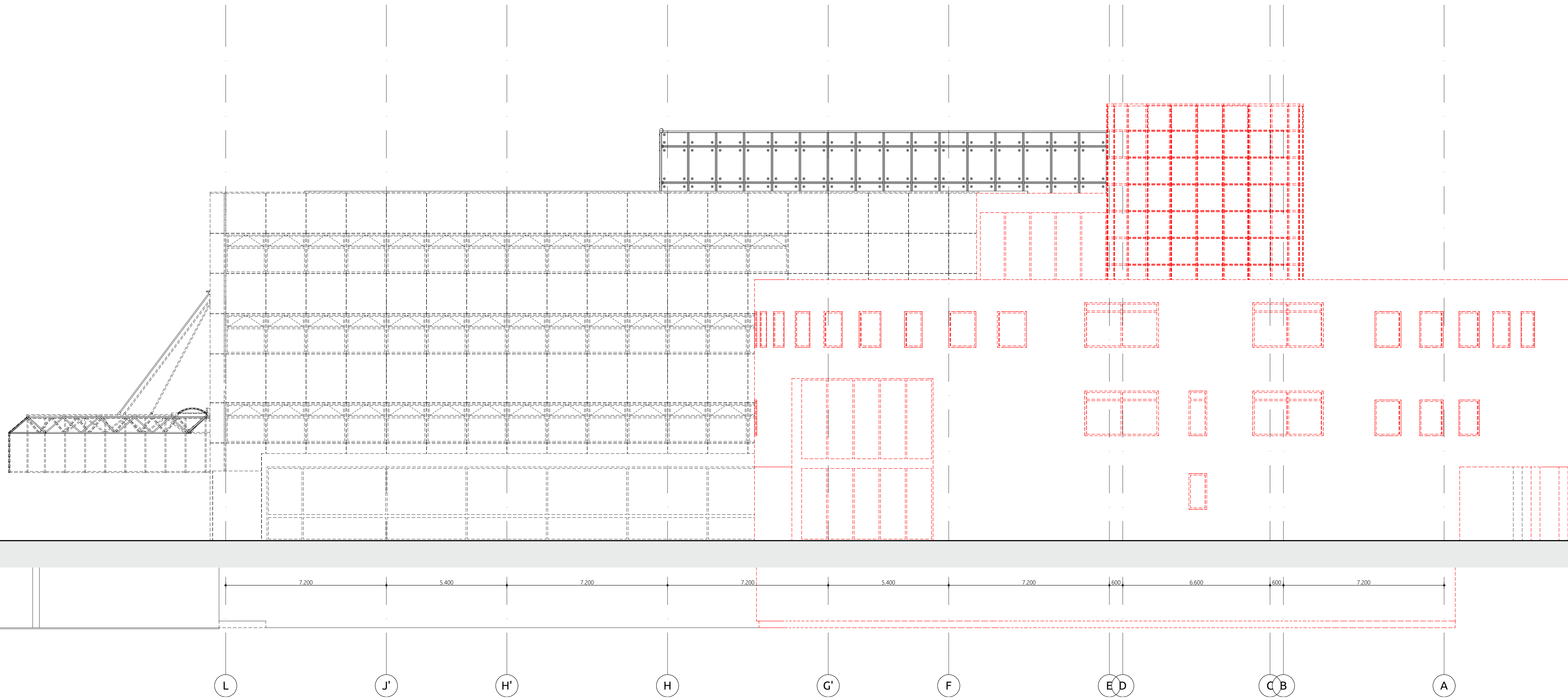
Noordgevel
