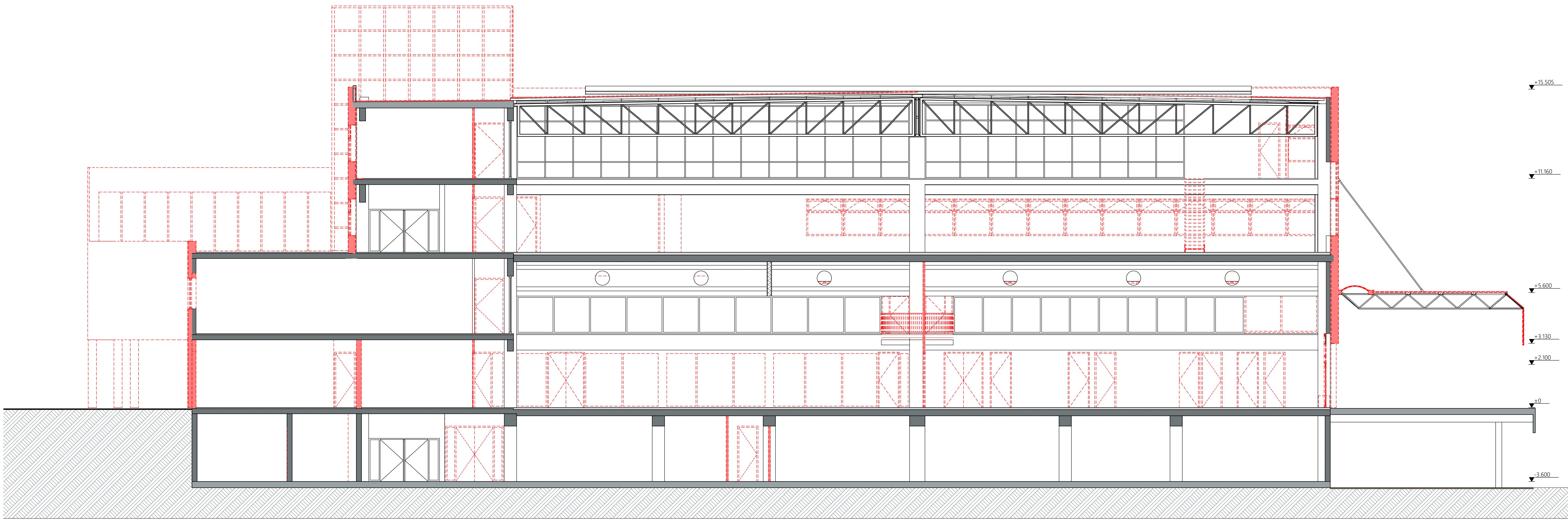
Doorsnede D-D
