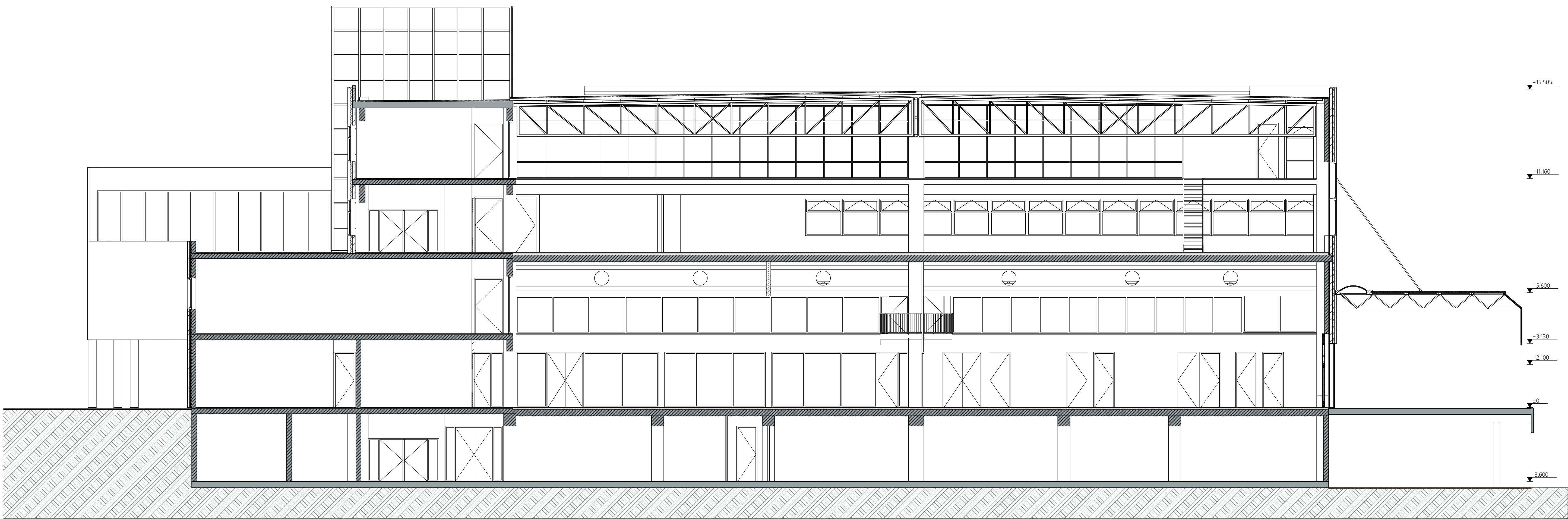
Doorsnede D-D
