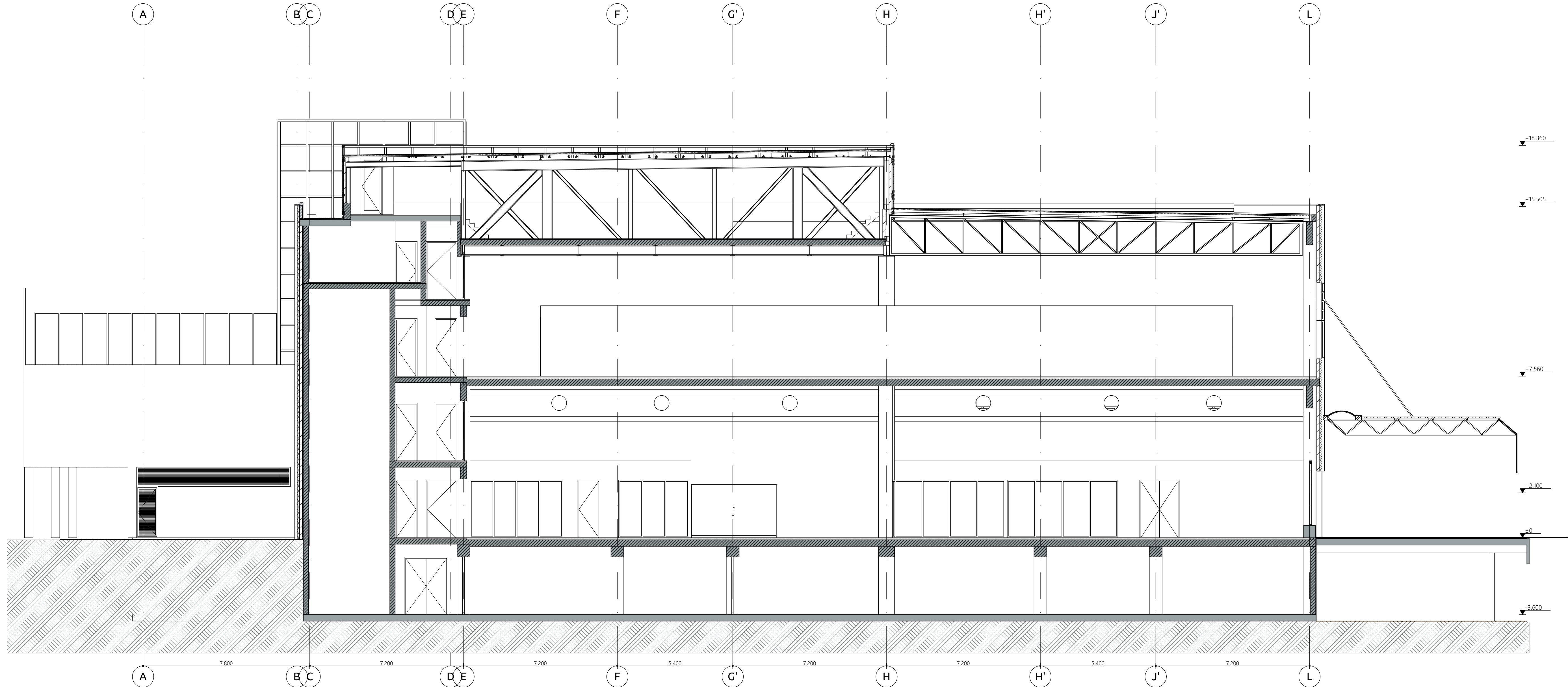
Doorsnede A-A
