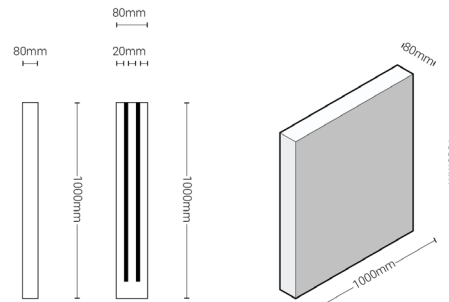
ZIJAAANZICHT
