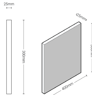
ZIJAAANZICHT
