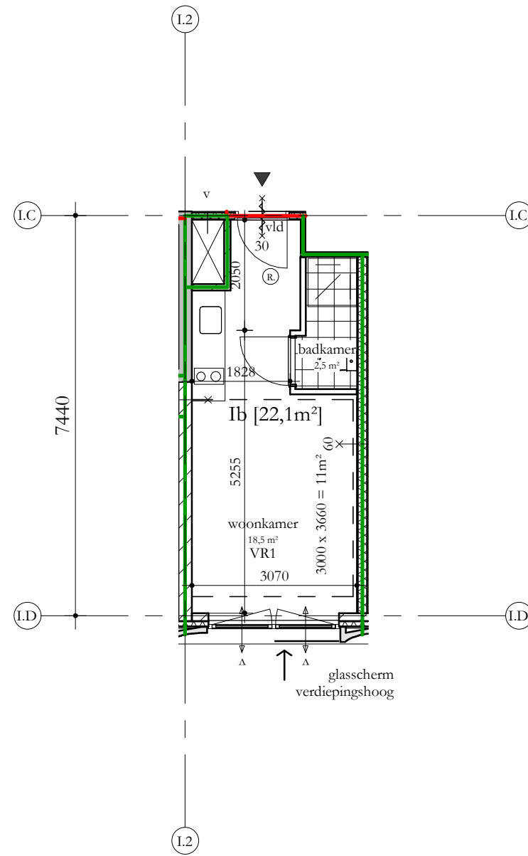
Type Ib 1 : 100
