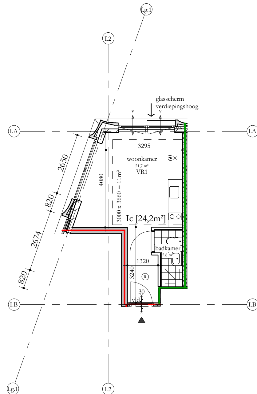
Type Ic 1 : 100
