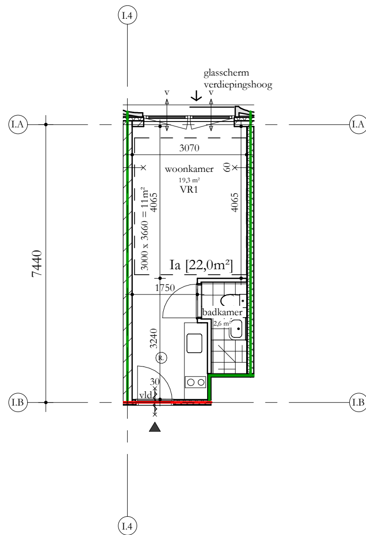
Type Ia 1 : 100
