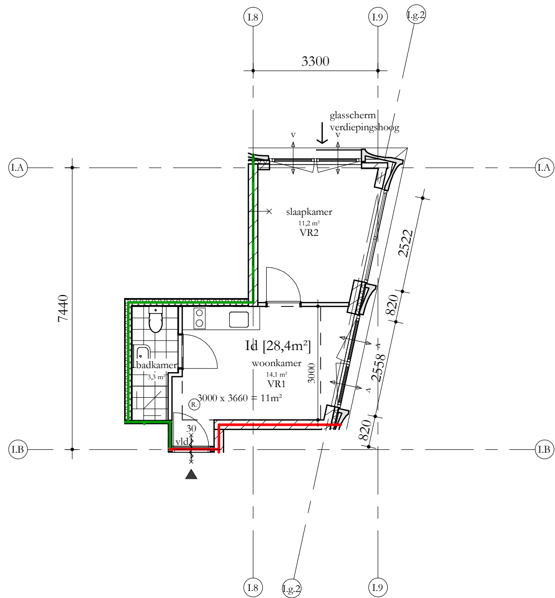
Type Id 1 : 100
