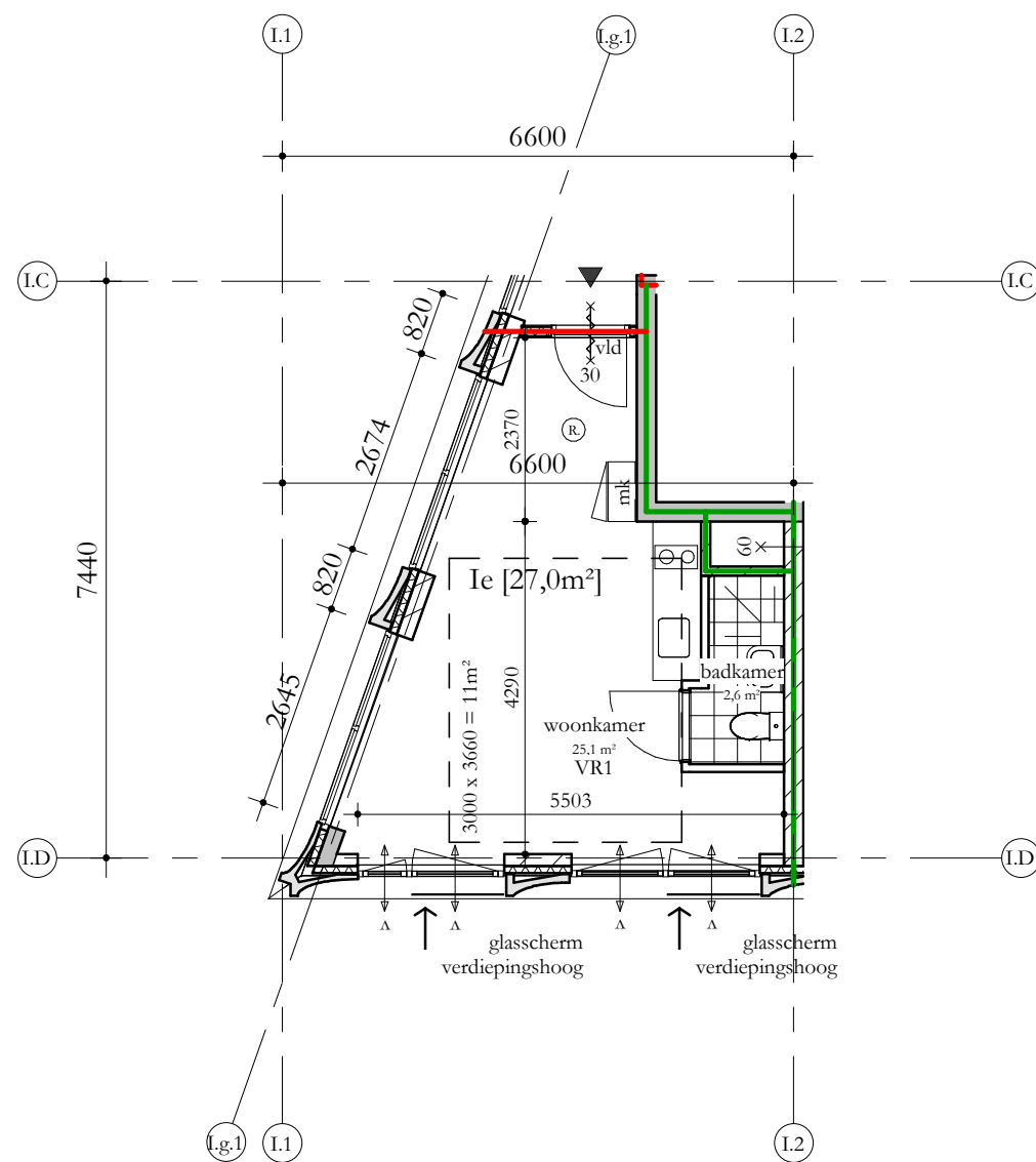
Type Ie 1 : 100
