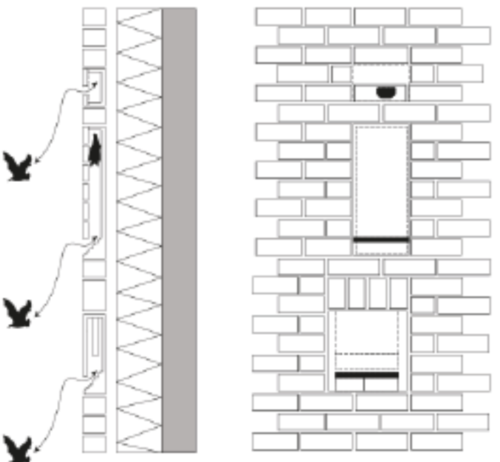
INBOUWKASTEN
