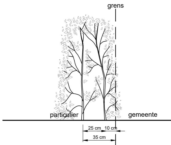
Dwarsprofiel
