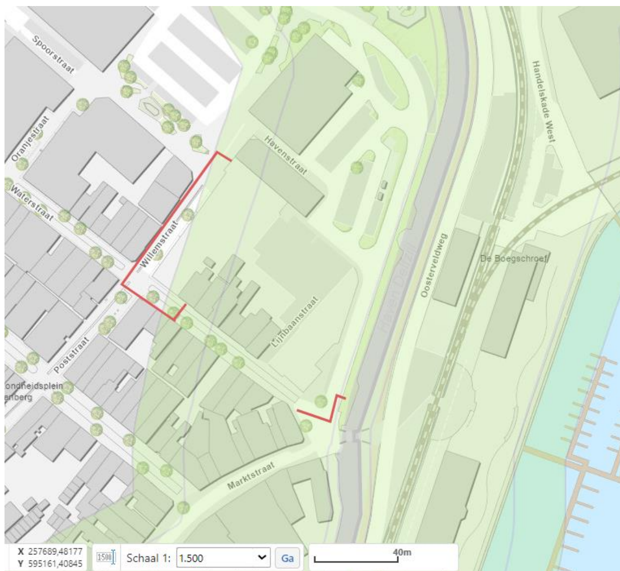
Figuur 1: Schematische tekening van de werkzaamheden. De rode lijnen geven globaal de locatie weer van de aan te leggen coax kabels.
