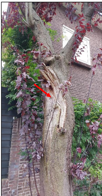
In de stam zijn verschillende mechanische defecten aanwezig, uitgescheurde tak, holte en rotting
