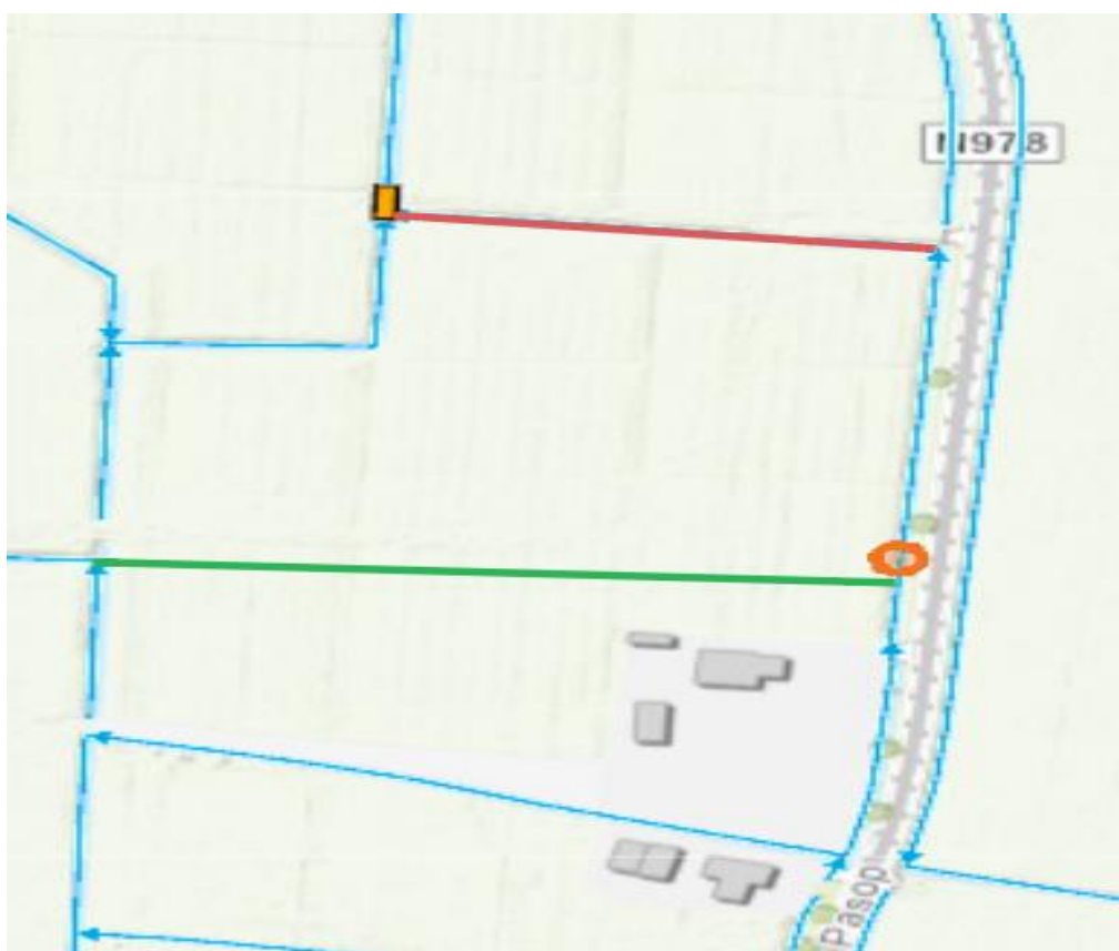
Figuur 1: Weergave te dempen sloot (rode lijn), te graven sloot met open verbindingen op aangrenzende sloten (groene lijn), nieuwe dam met duiker (oranje cirkel).
