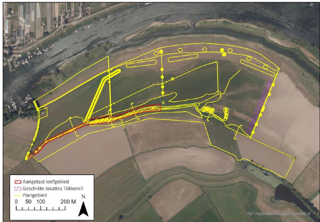
Figuur 2. Langs de oostkant van het projectgebied worden minimaal twee takkenrillen aangelegd als voortplantings- of rustplaats voor klein marterachtigen.
