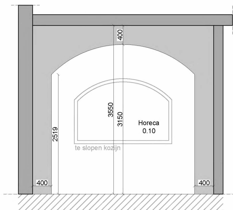
Doorsnede / aanzicht doorbraak
