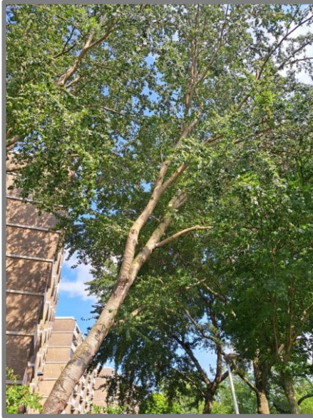
Fig. 1: De boom staat scheef en vertoont aan de stam en de kroon geen tekenen van 'oprichten' (links). Dit betekent dat de boom recentelijk is verzakt en instabiel is. Aan de trekzijde van de stamvoet is de grond wat omhoog gekomen, maar door de dichte begroeiing zijn er geen grondscheuren waargenomen (rechts).
